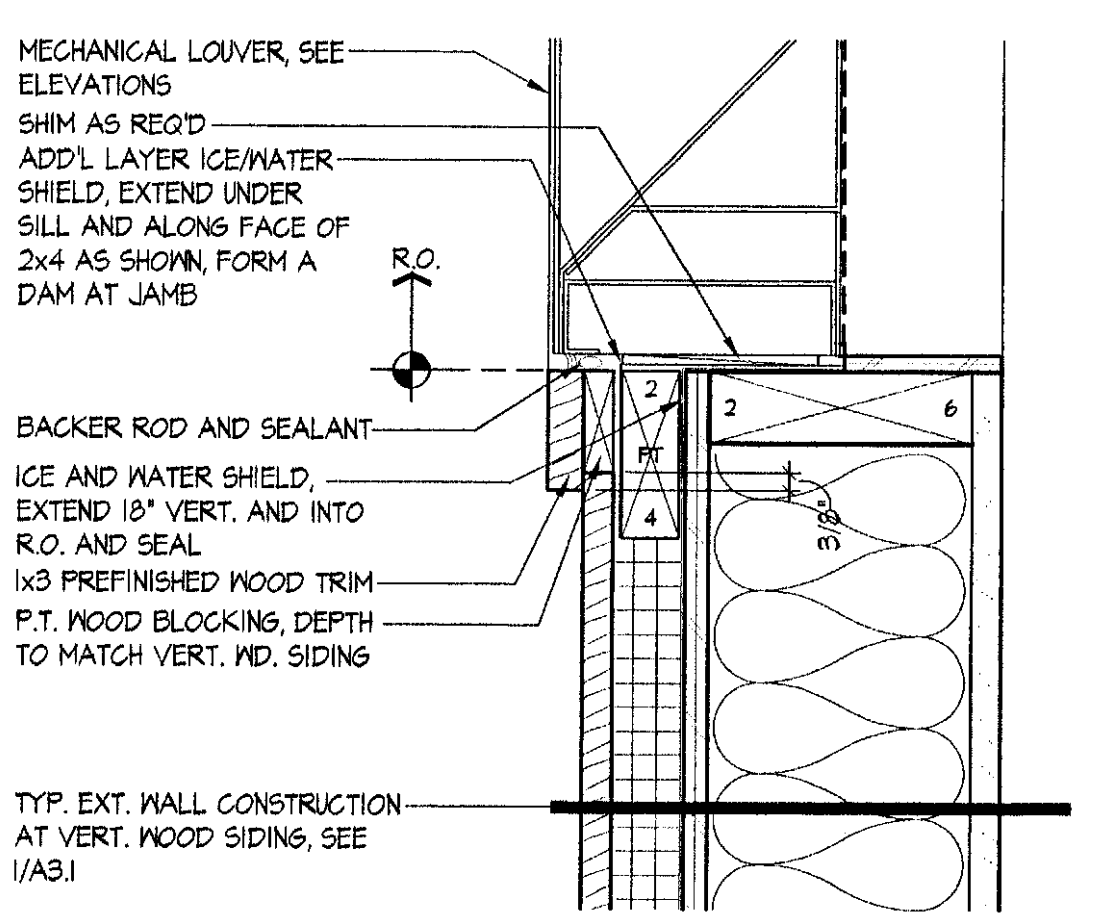
6 LOUVER SILL DETAIL SCALE: 3" = 1'-0" 2003_DTL-LOUVER
