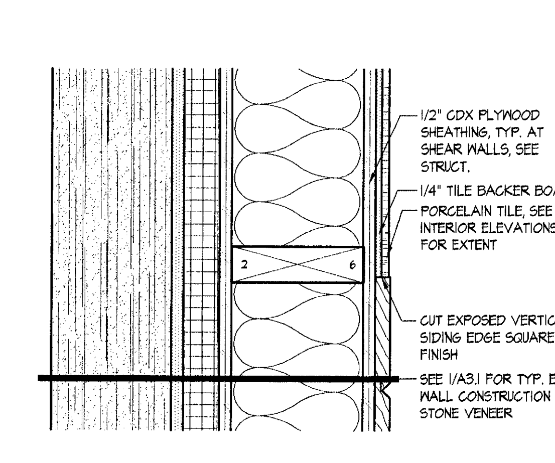
8 HORIZ. TILE TRANS./SHEAR WALL SCALE: 3" = 1'-0" 2003_DTL-TILE01
