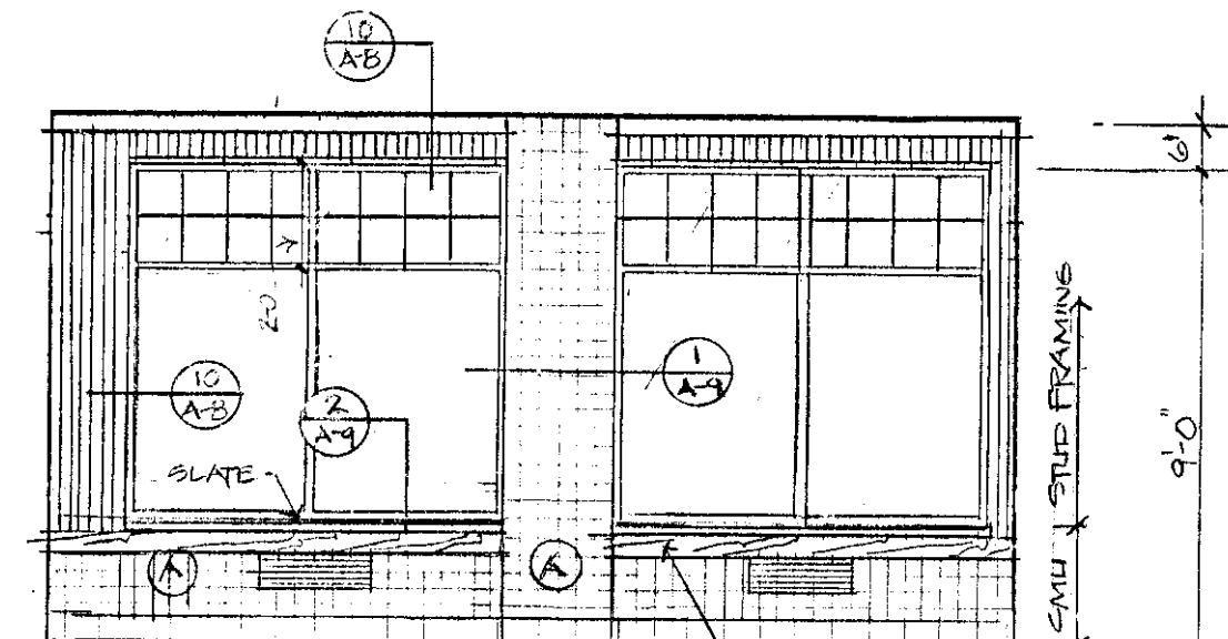
04 Foyer 100A Scale: 1/4" = 1'-0"
