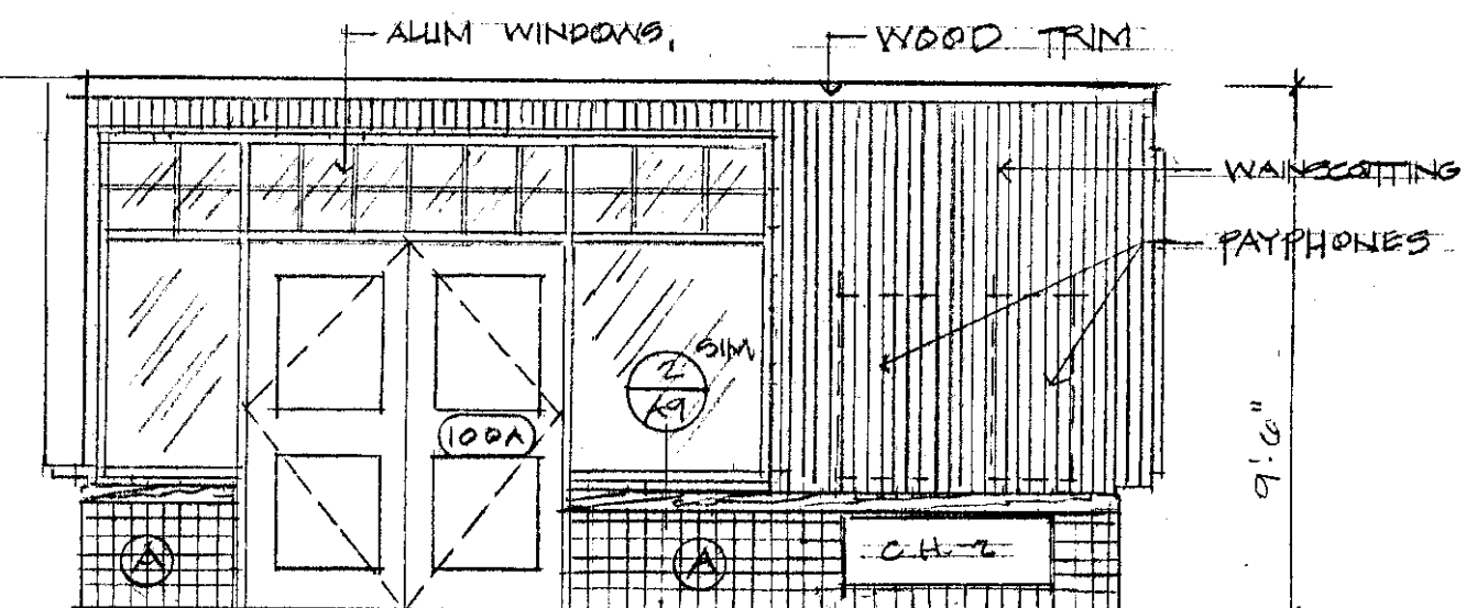
09 Entry Vestibule Scale: 1/4" = 1'-0"
