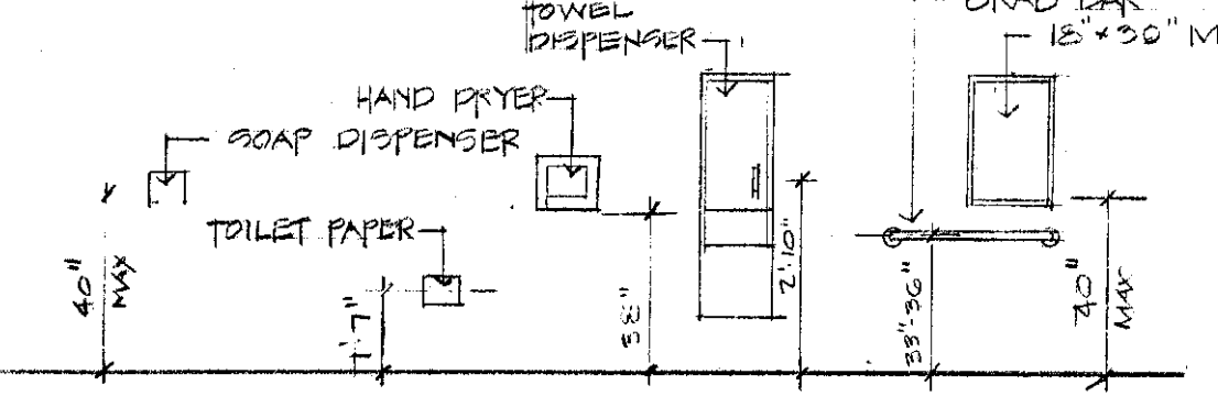
08 Restroom 101 Scale: 1/4" = 1'-0"
