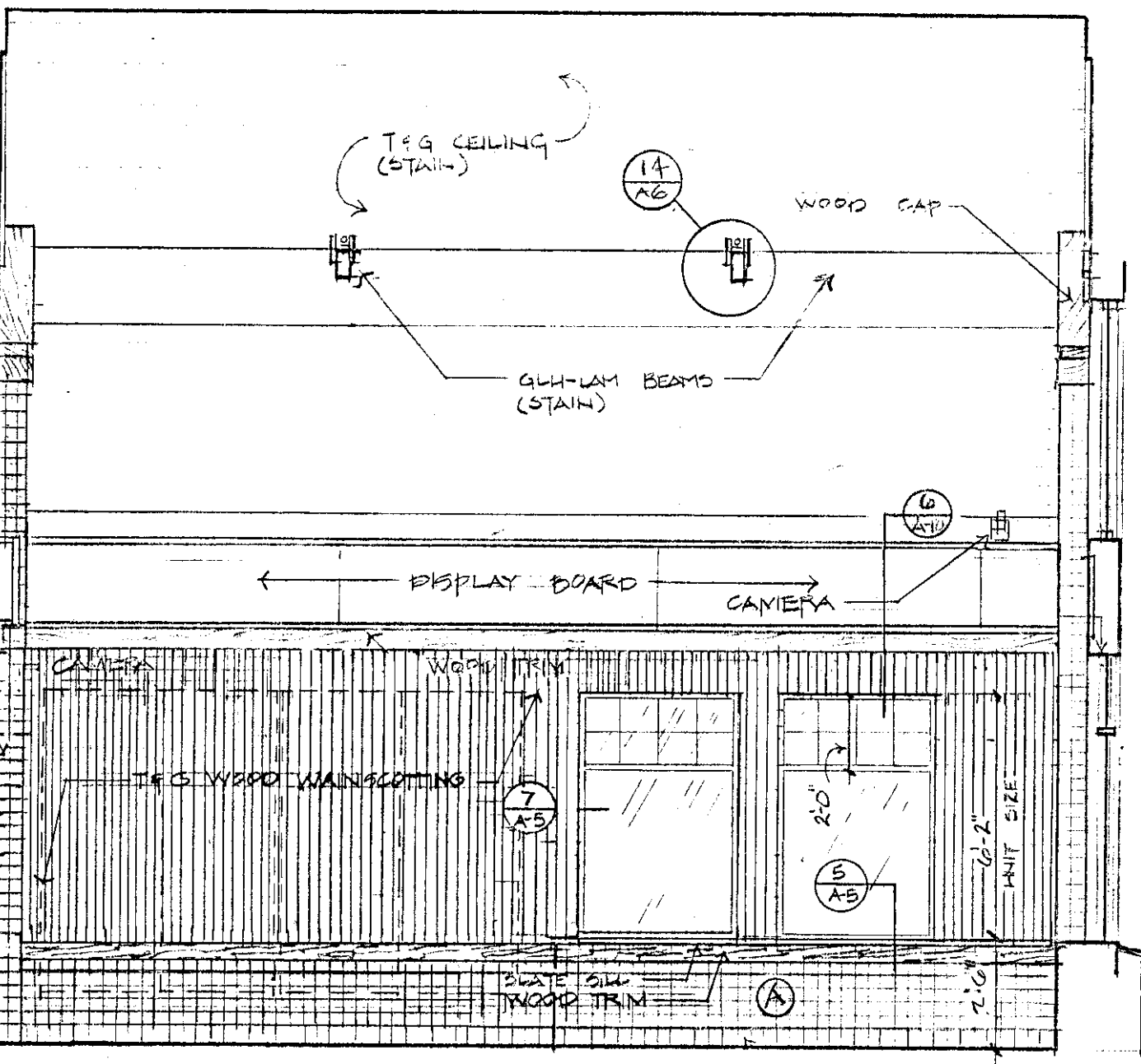
03 Foyer 100A Scale: 1/4" = 1'-0"
