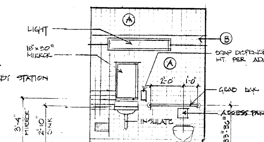
06 Restroom 101 Scale: 1/4" = 1'-0"
