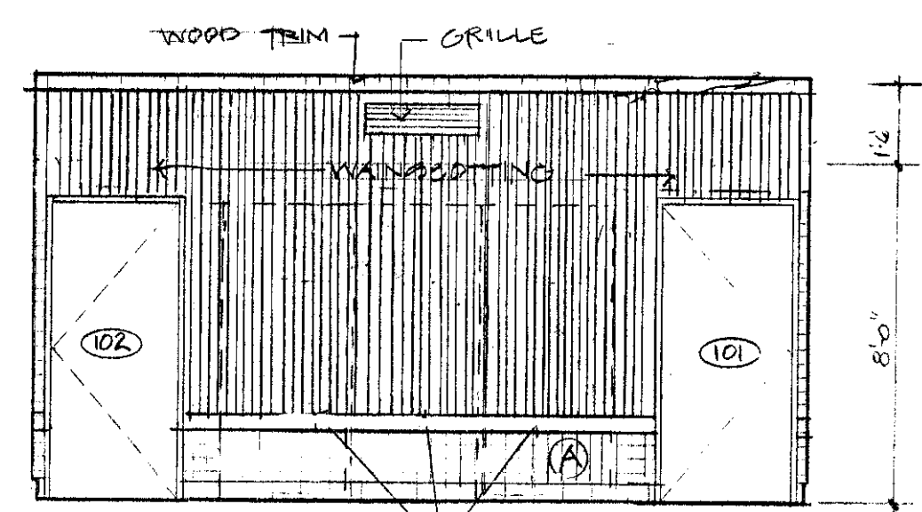
02 Foyer 100A Scale: 1/4" = 1'-0"
