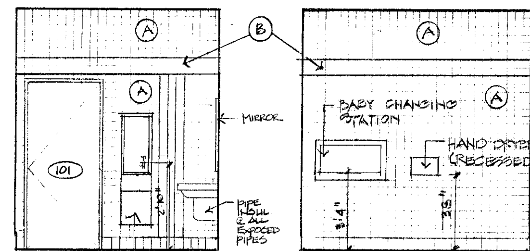
07 Restroom 101 Scale: 1/4" = 1'-0"
