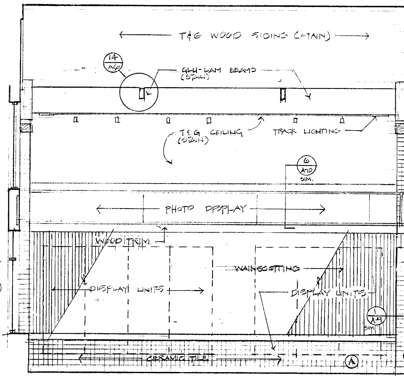
13 Display 105 Scale: 1/4" = 1'-0"
