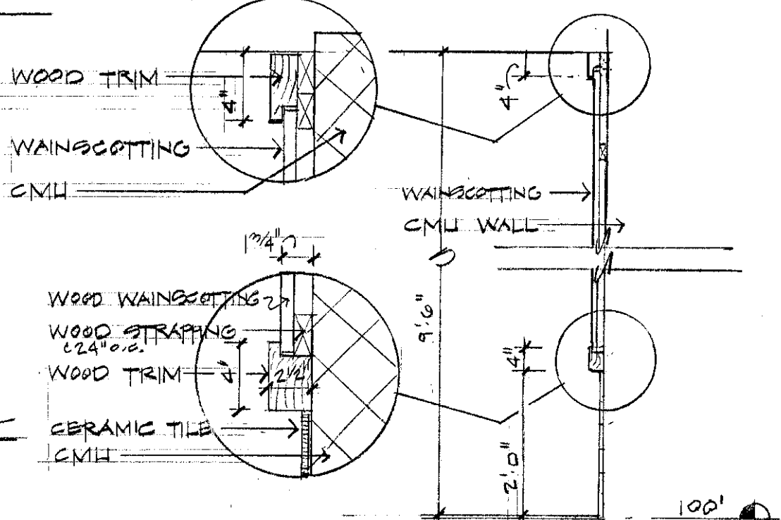
17 Wall Detail Scale: 1/2" = 1'-0"
