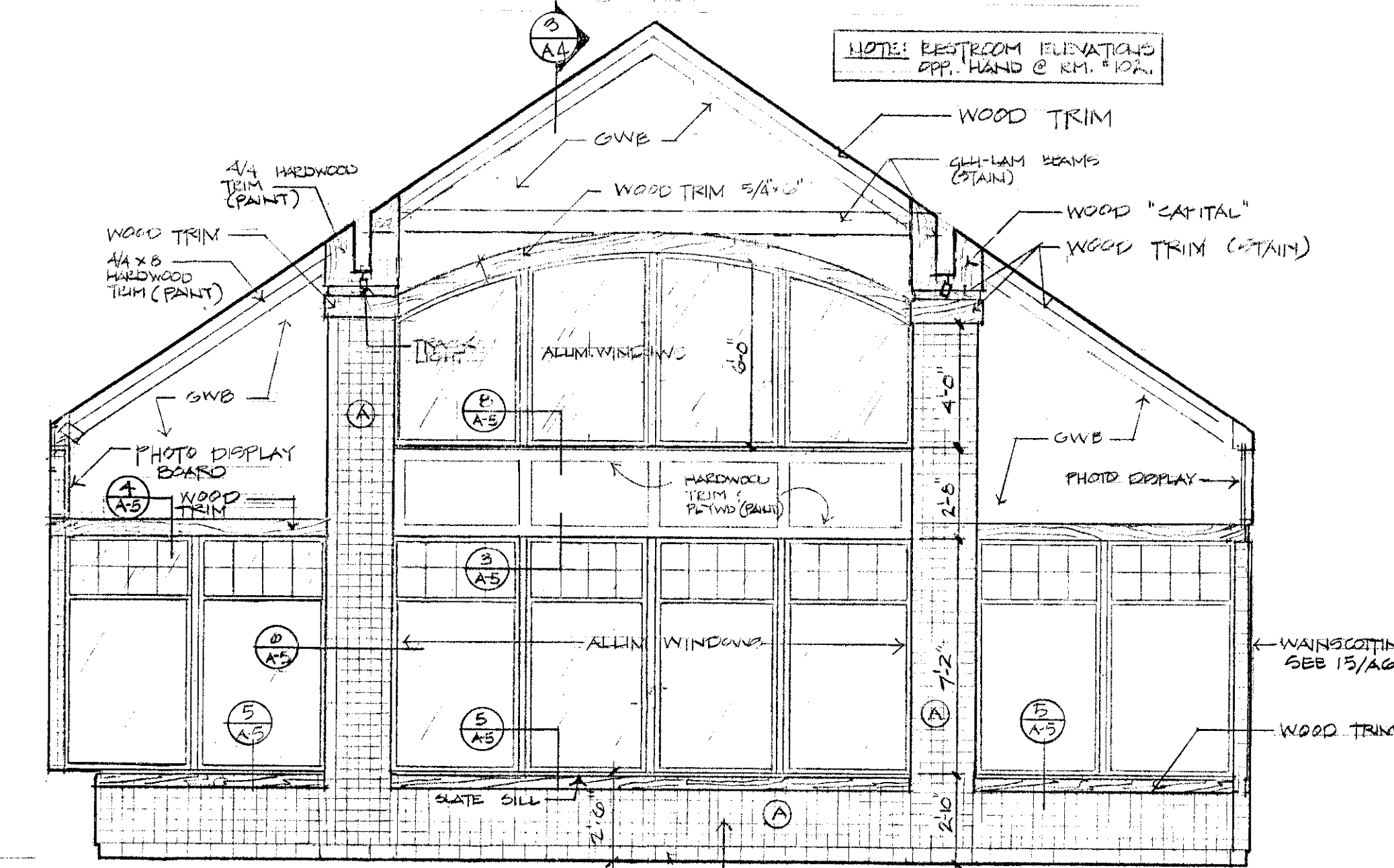
11 Display 105 Scale: 1/4" = 1'-0"
