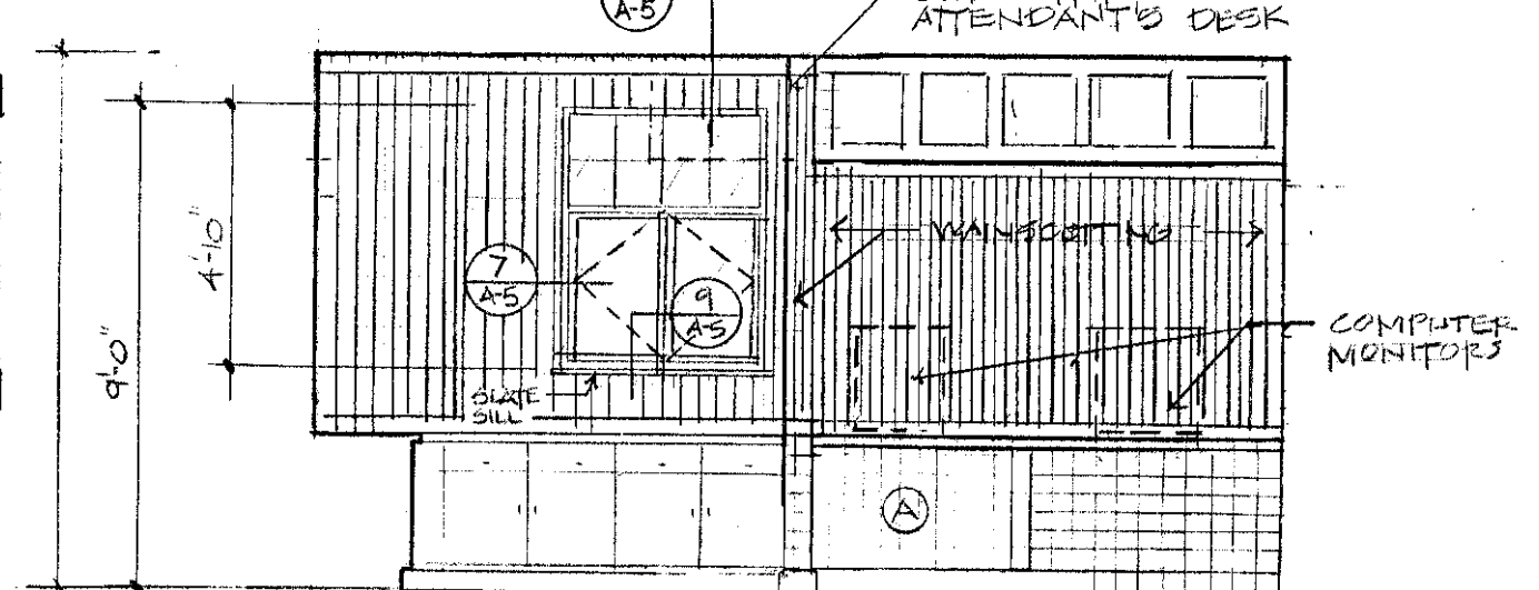
15 Attendant 103 Scale: 1/4" = 1'-0"
