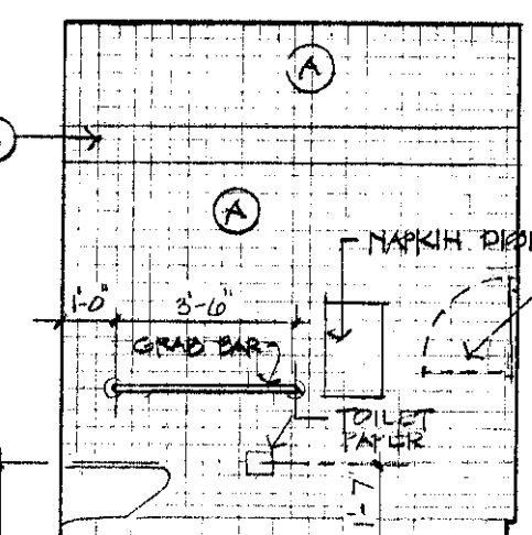
05 Restroom 101 Scale: 1/4" = 1'-0"
