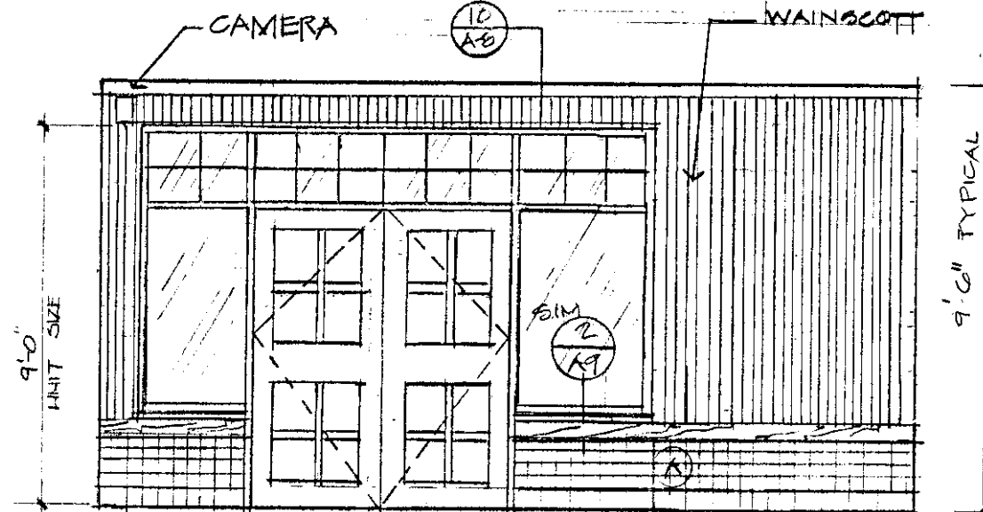
03 Foyer 100A Scale: 1/4" = 1'-0"
