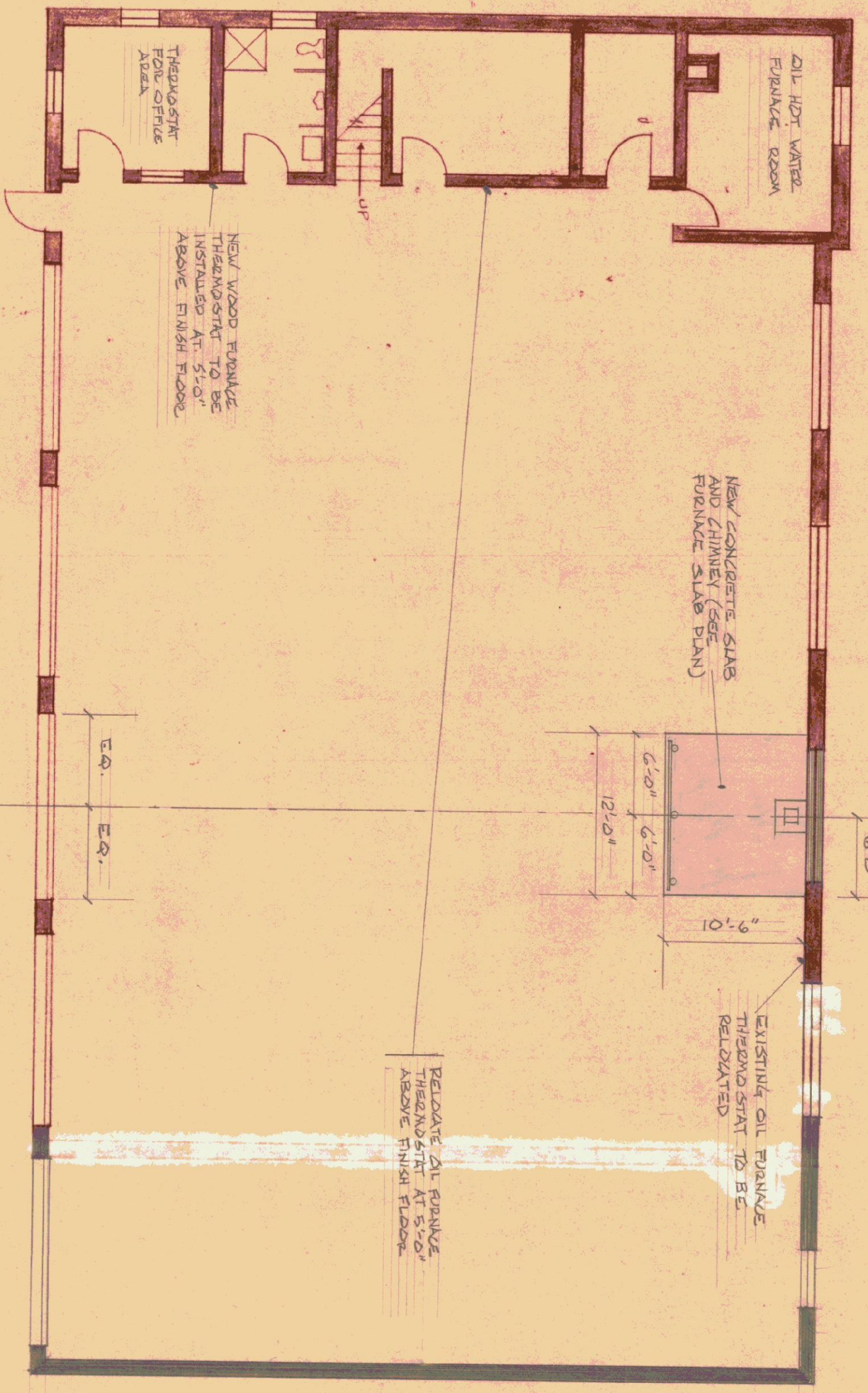
FLOOR PLAN SCALE: 1/8" = 1'-0"
