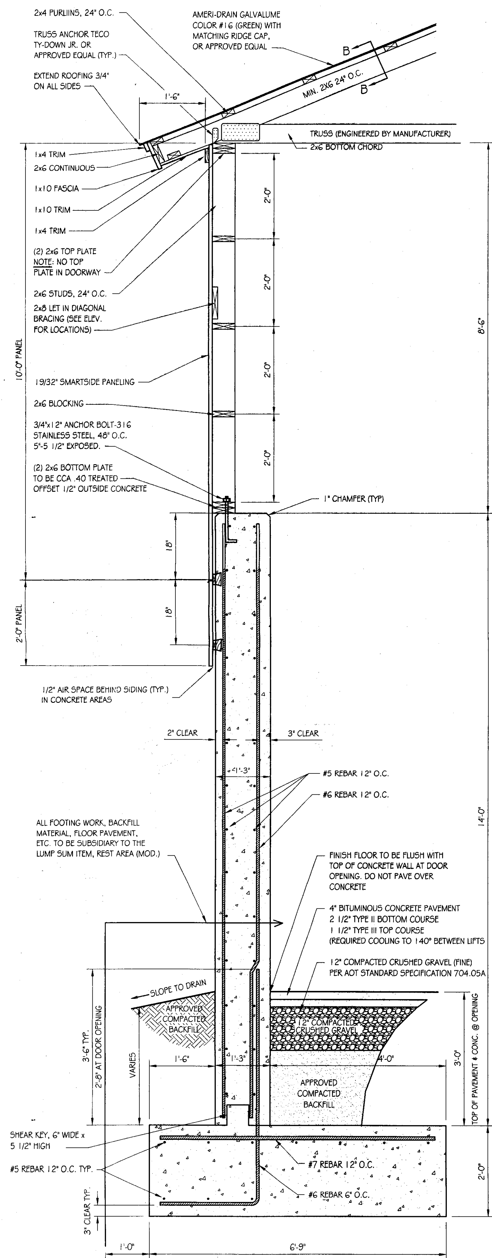
A A2 WALL SECTION SCALE: 3/4" = 1'-0"
