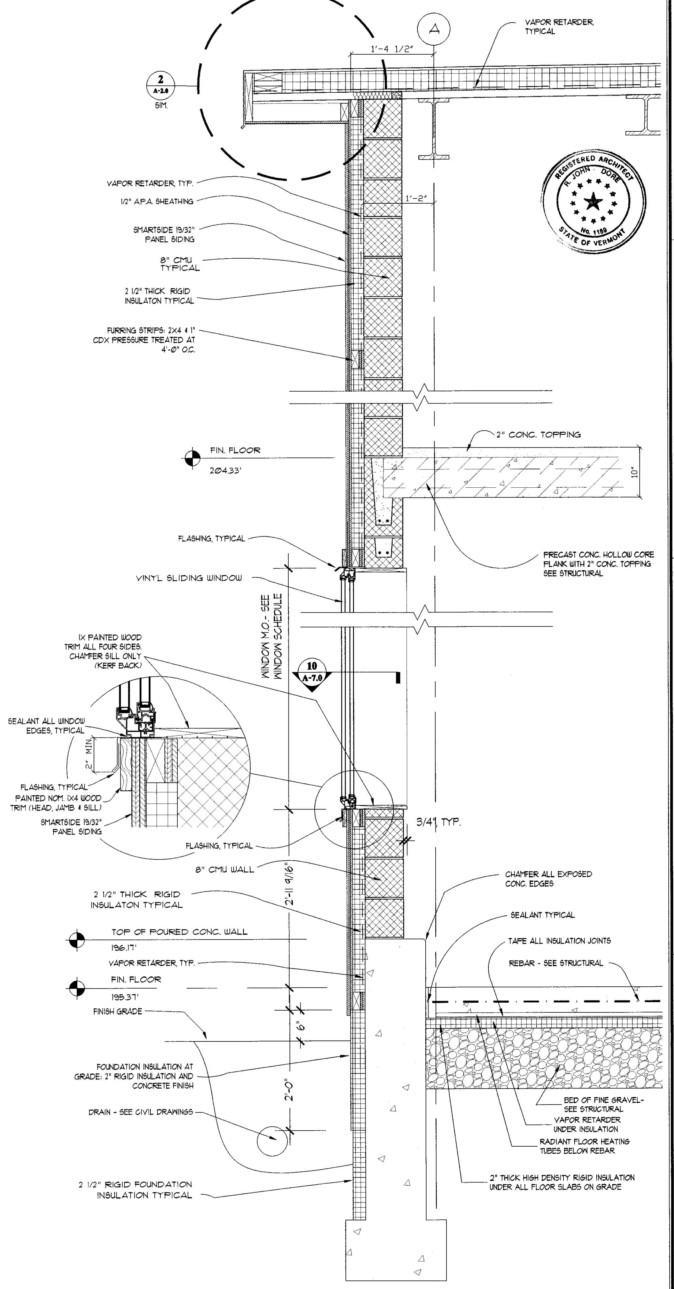
6 WALL SECTION SCALE: 1" = 1'-0"
