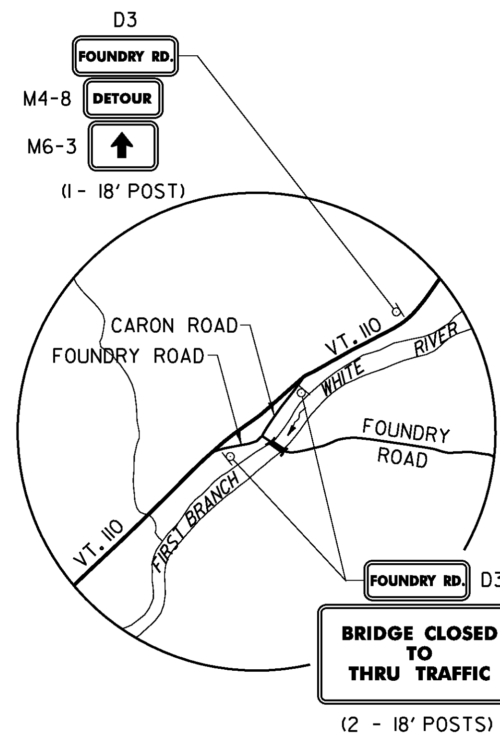
DETAIL 2 SCALE: 1" = 500'
