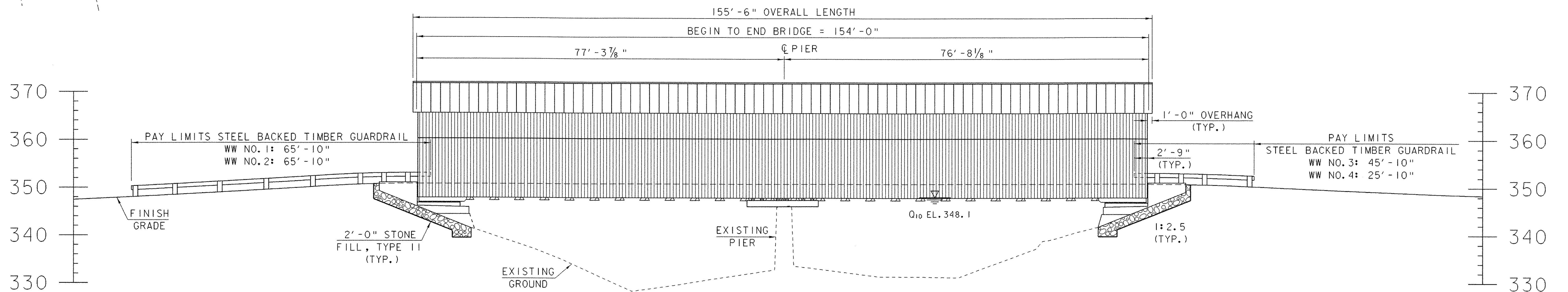
ELEVATION 10 0 10 SCALE: 1" = 10'-0"
