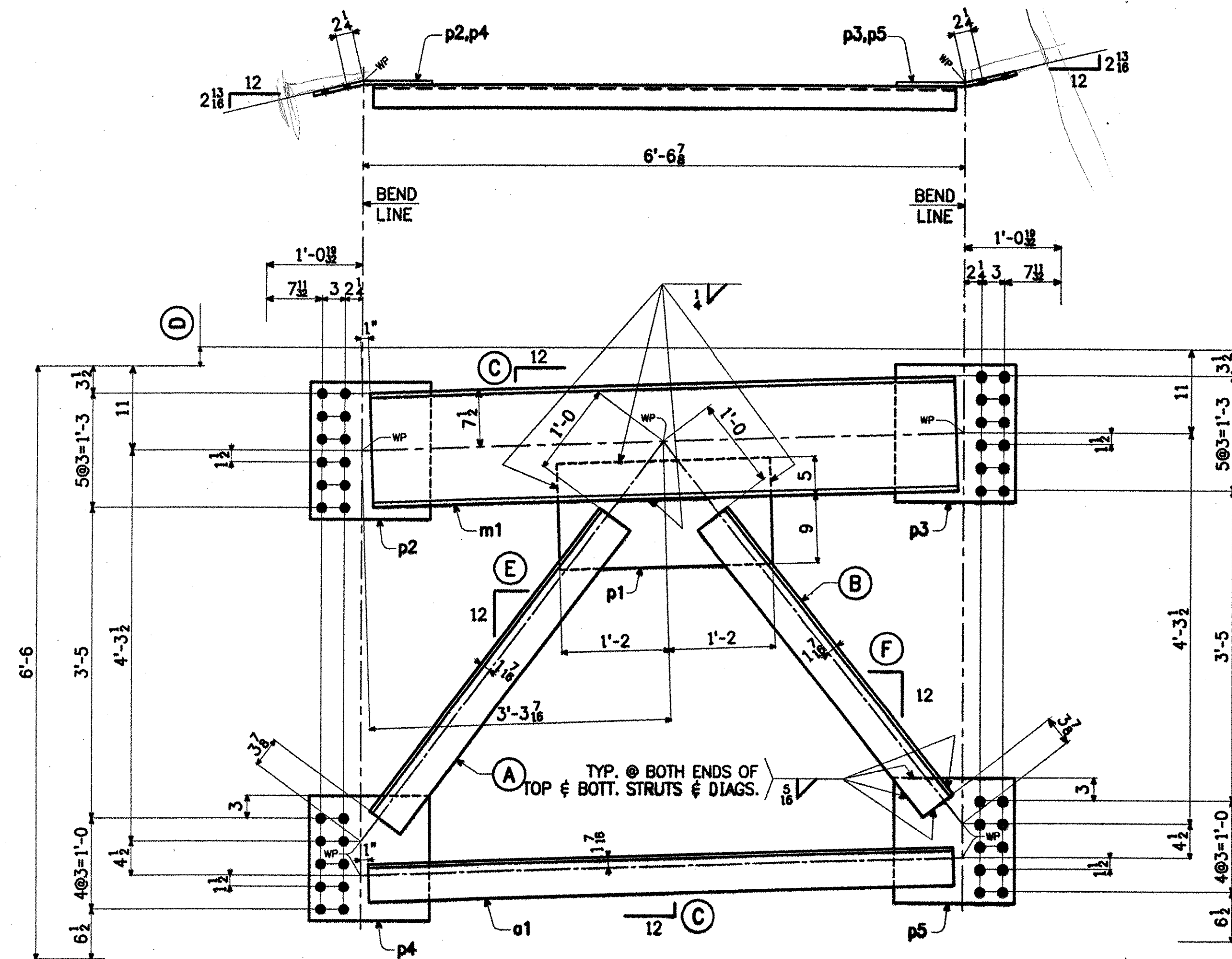
ABUT. CROSSFRAMES
