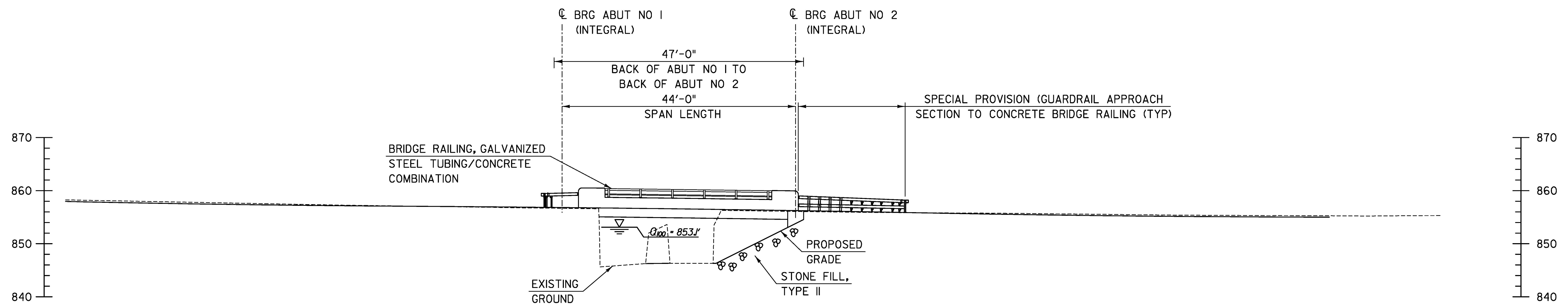
ELEVATION SCALE: 1" = 10'-0"
