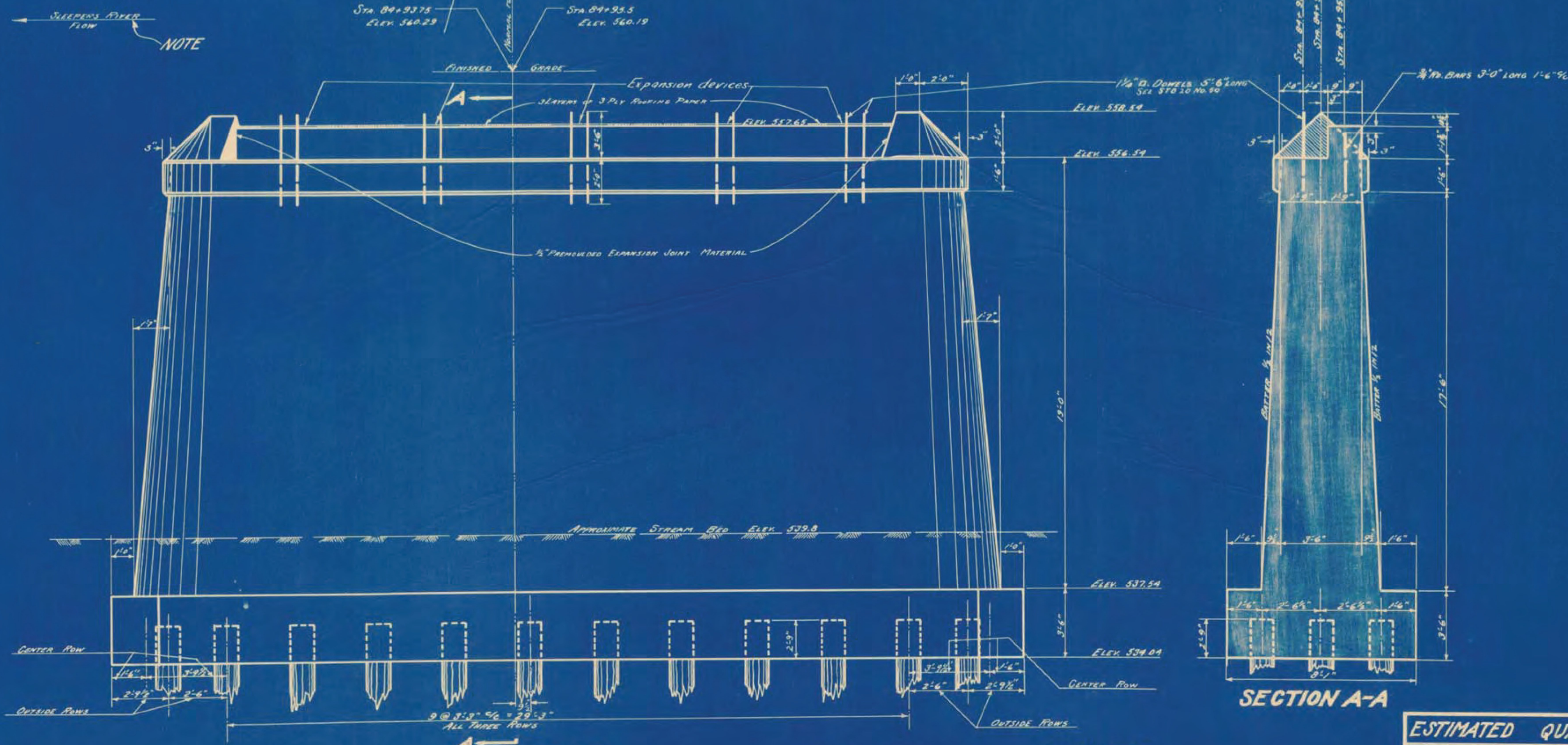
ELEVATION
