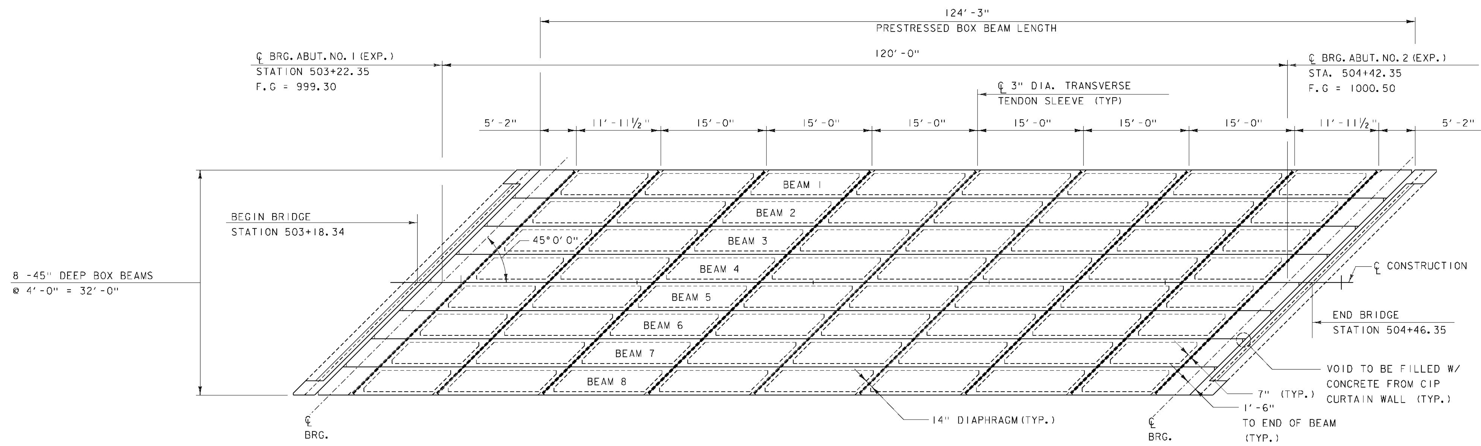
FRAMING PLAN SCALE: 1/8" = 1'-0"
