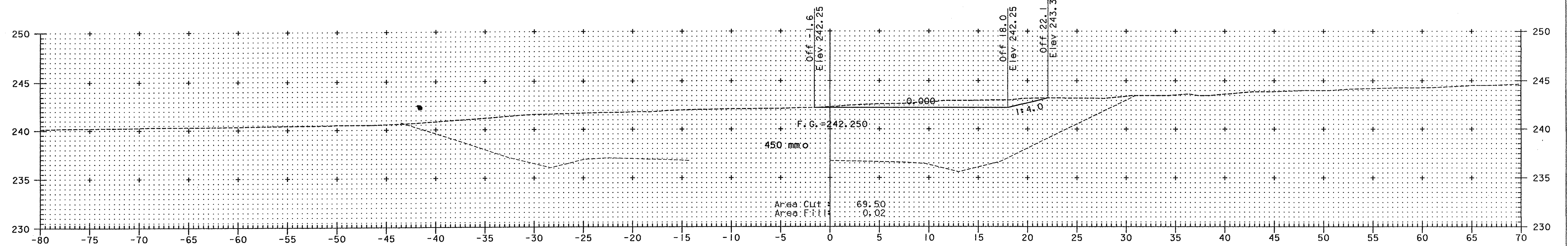
B 1+580 Volume Cut : 4287.53 Volume Fill : 0.20
