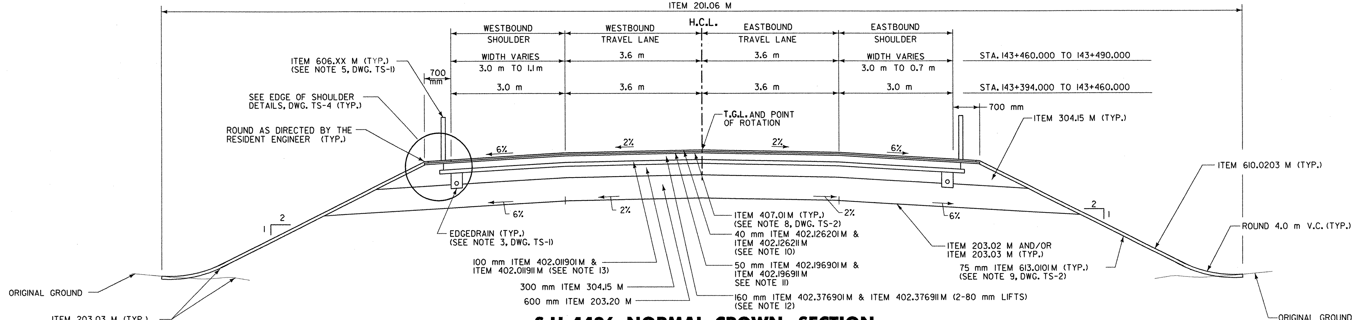
S.H. 1426 NORMAL CROWN SECTION N.T.S. STA. 143+394.000 TO 143+490.000
