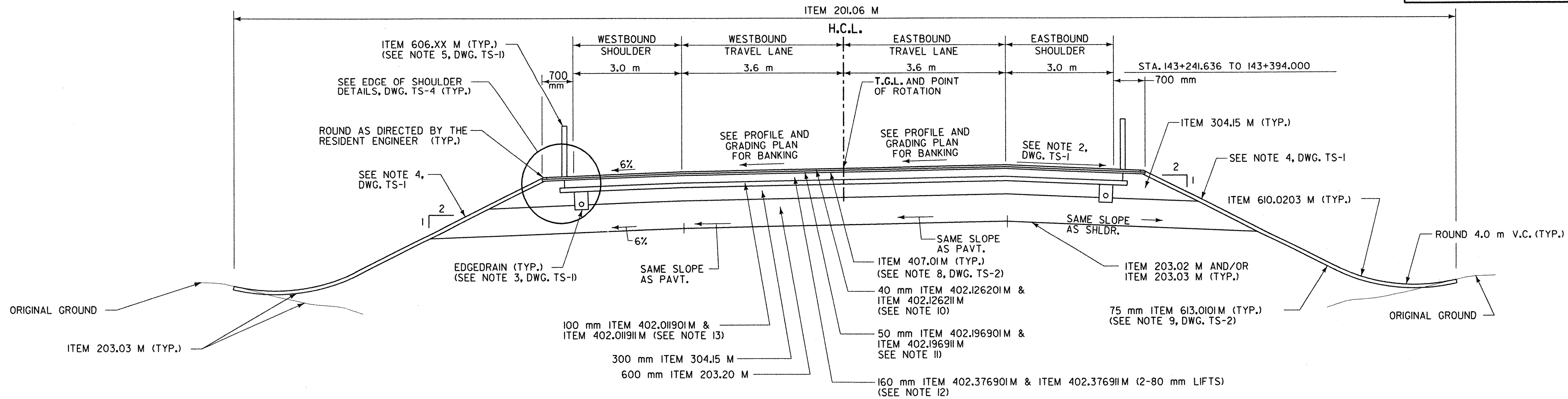
S.H. 1426 BANKED SECTION N.T.S. STA. 143+241.636 TO 143+394.000
