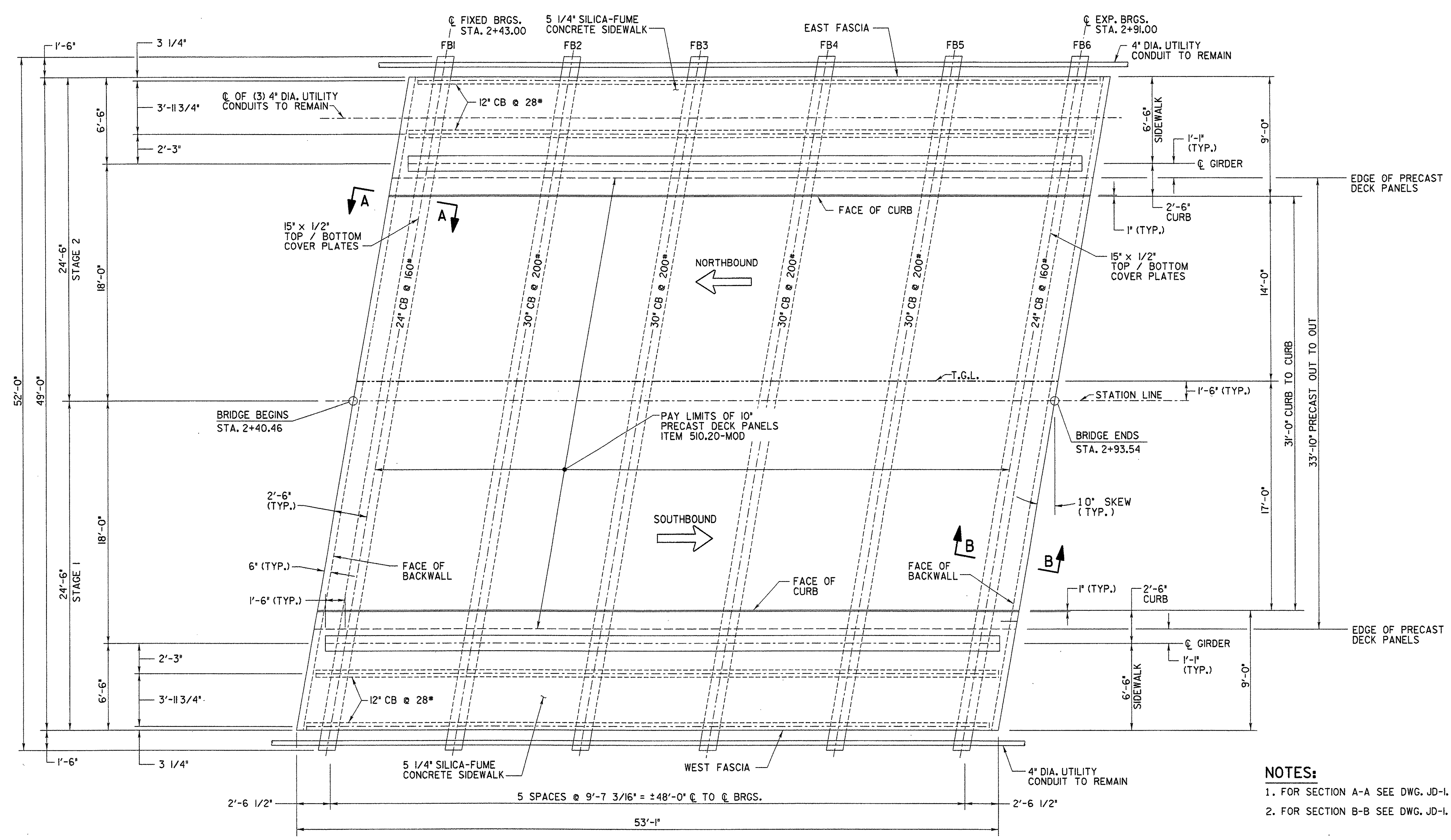
PLAN SCALE: 1/4" = 1'-0"
