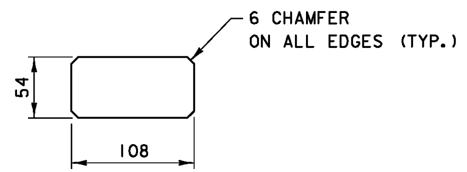
SECTION D-D
