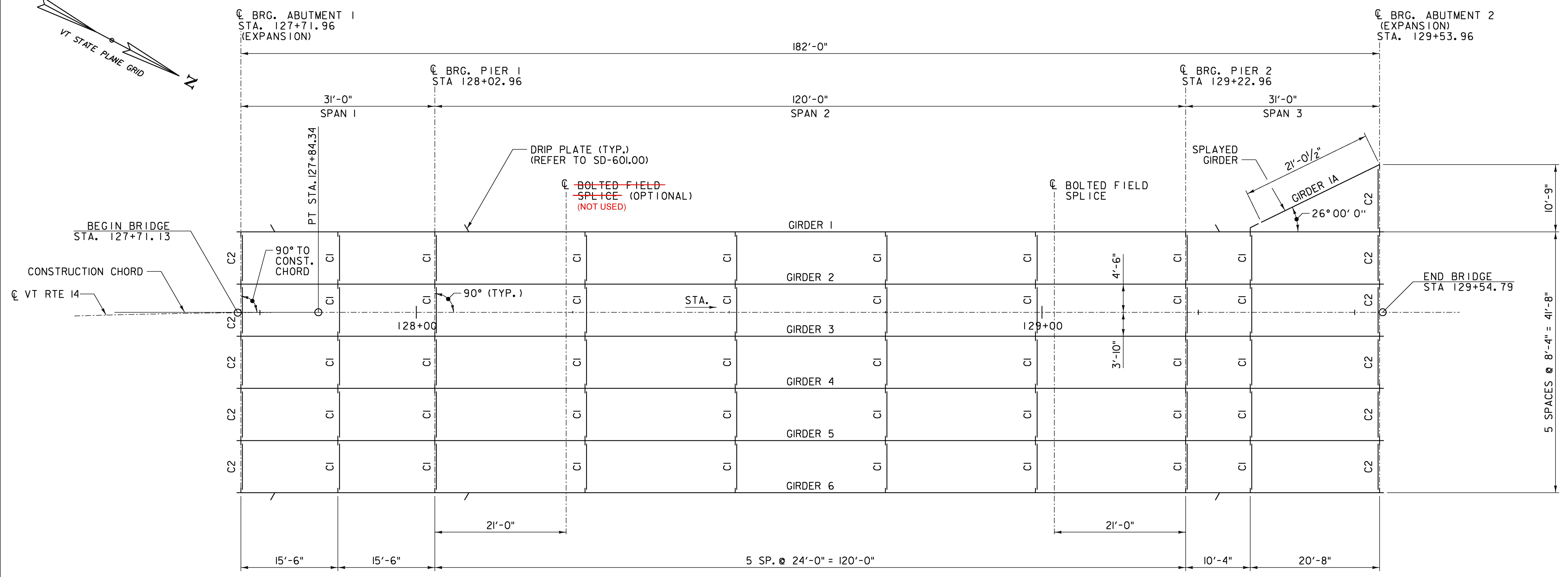
FRAMING PLAN SCALE: 1/8" = 1'-0"
