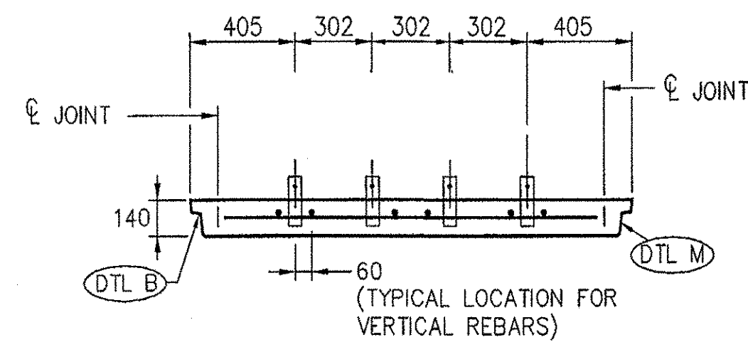
SECTION A-A FOR 4 T.S. PER LEVEL SCALE 1:20
