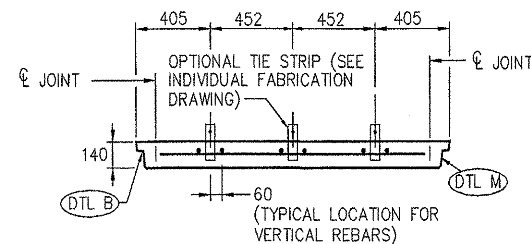
SECTION A-A FOR 2 OR 3 T.S. PER LEVEL SCALE 1:20
