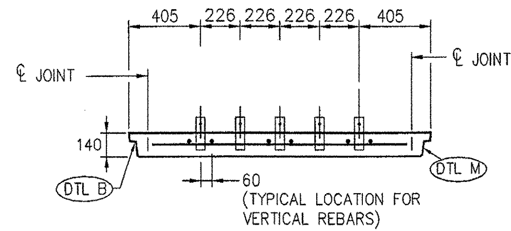
SECTION A-A FOR 5 T.S. PER LEVEL SCALE 1:20
