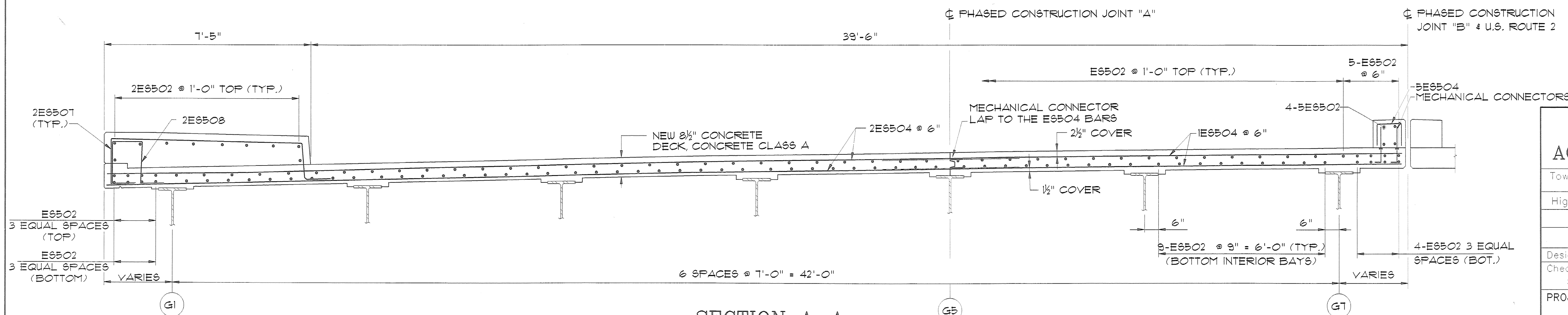
SECTION A-A SCALE: 1/2"=1'-0"
