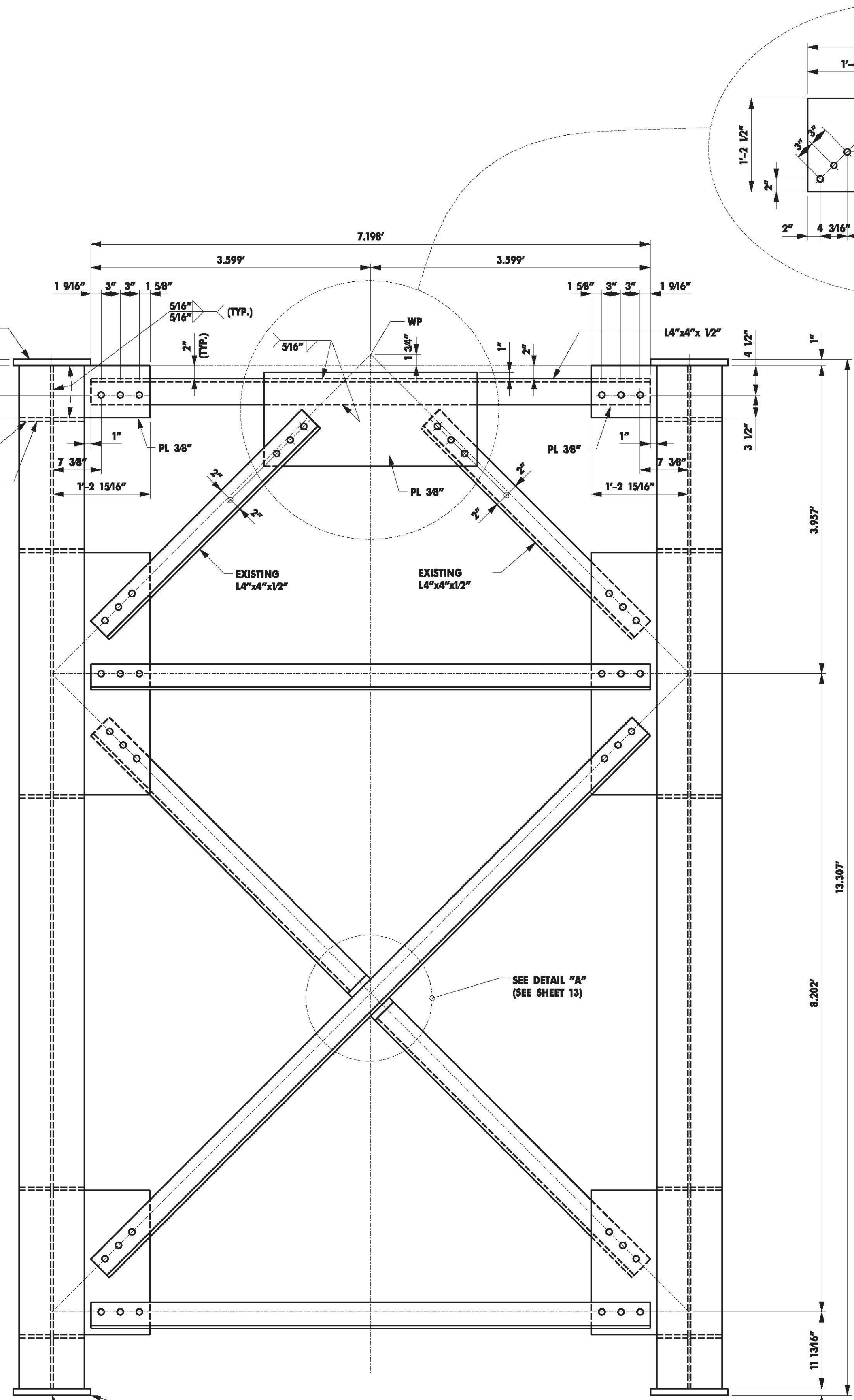
ELEVATION
