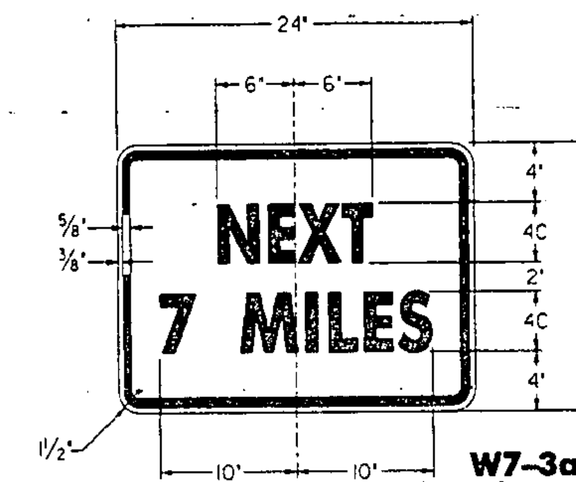
W7-3a
