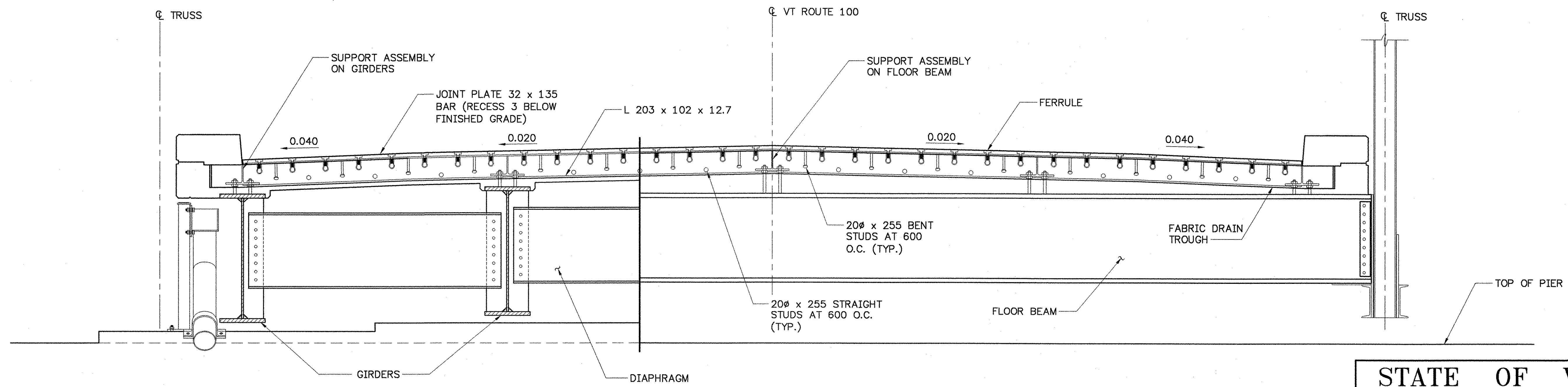
SECTION A-A SCALE 1:20
