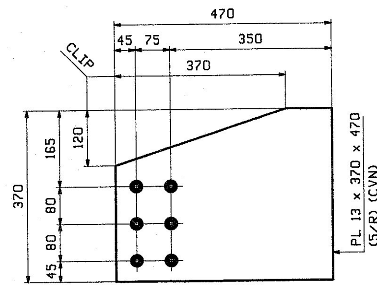
60 ~ GUSSET PL ~ mb BOTTOM
