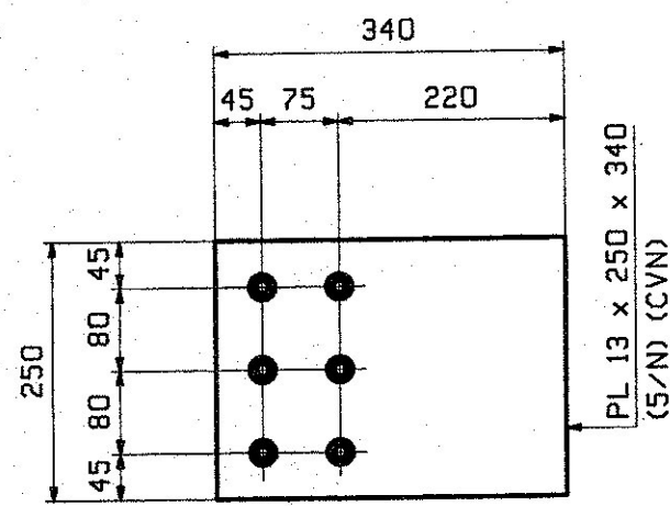
24 ~ GUSSET PL ~ mla ABUT. & PIER - TOP
