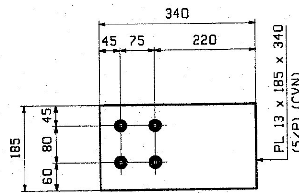
96 ~ GUSSET PL ~ md INT. CF - TOP
