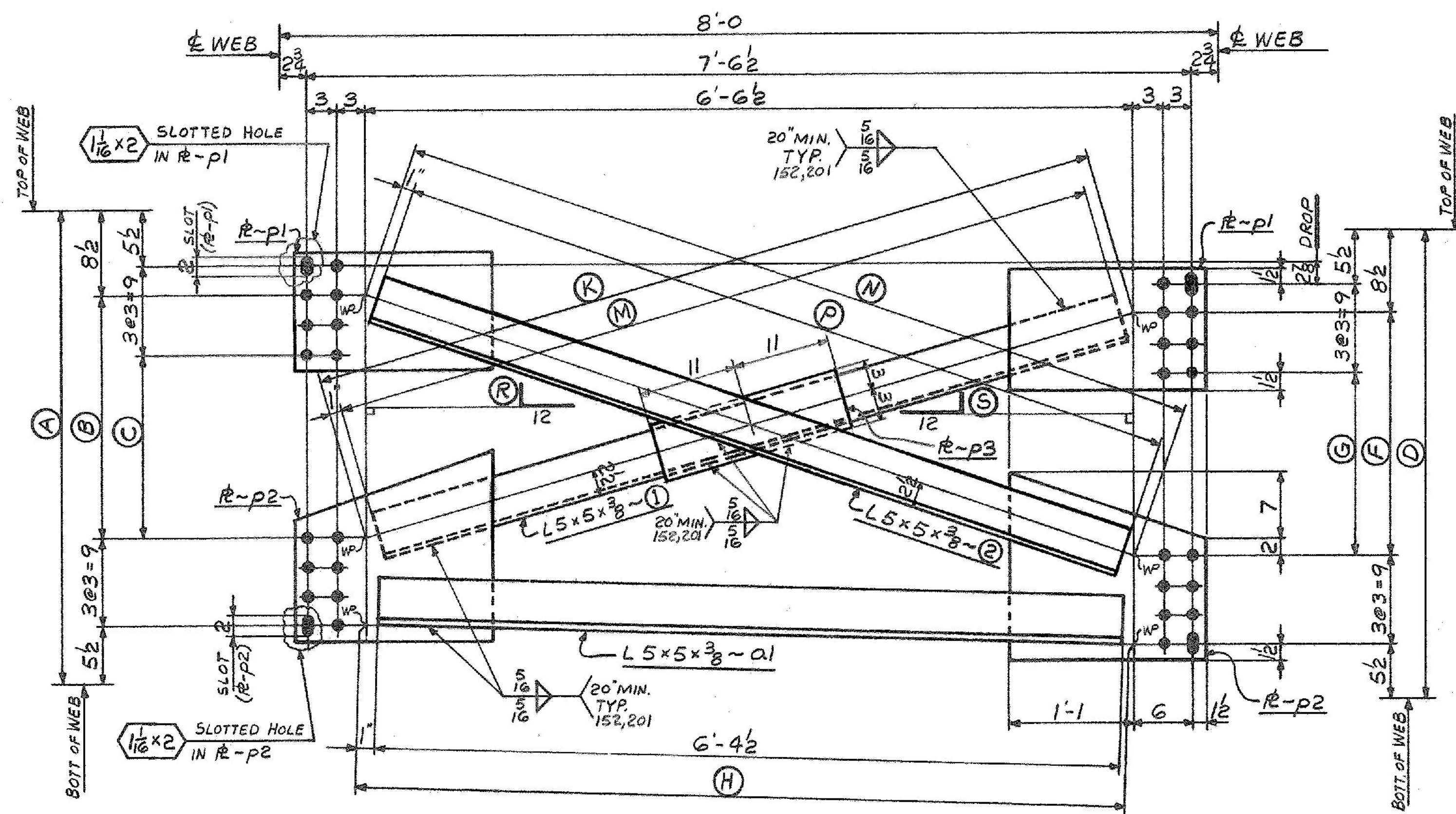
CROSSFRAMES
