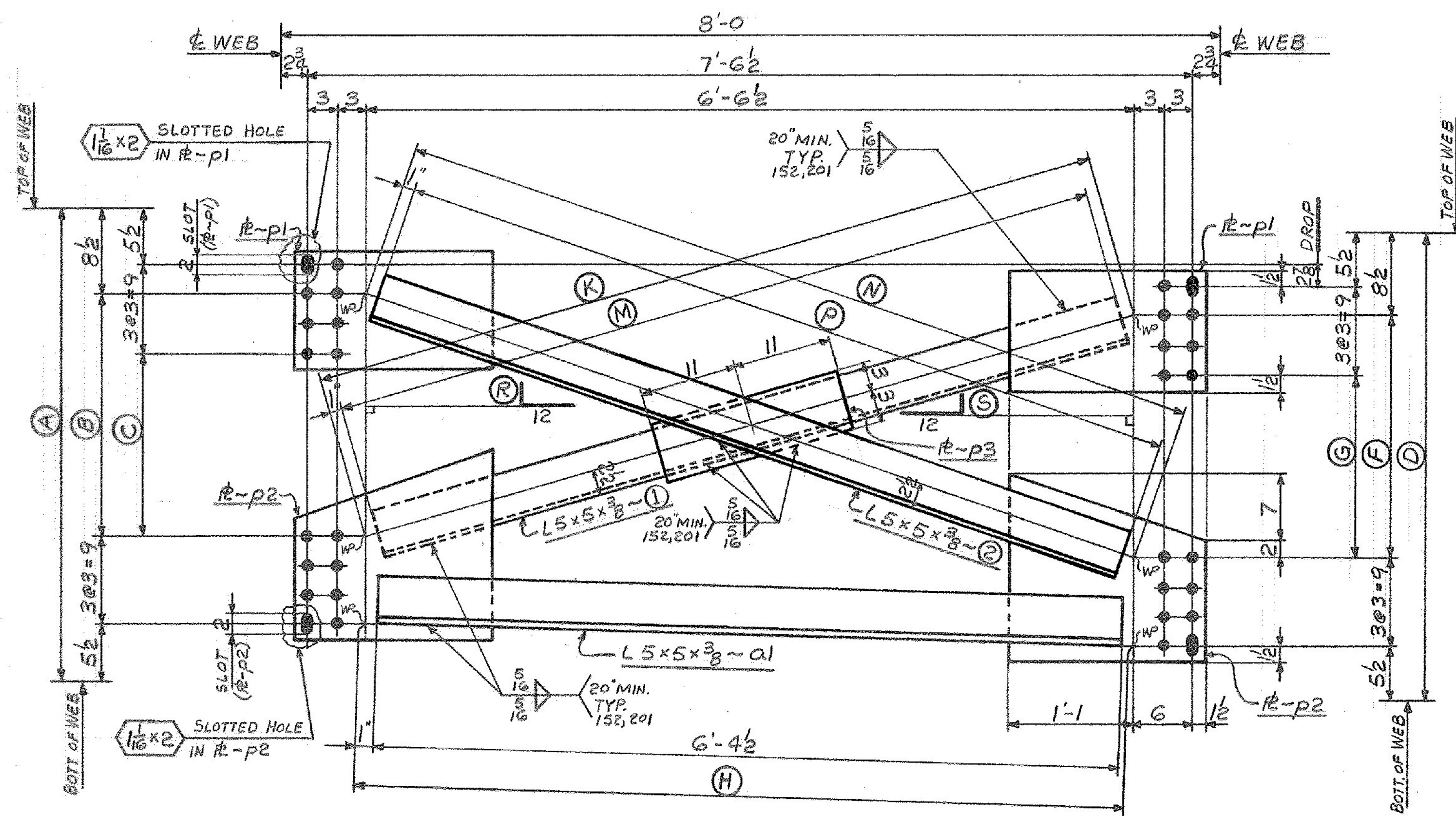
CROSSFRAMES
