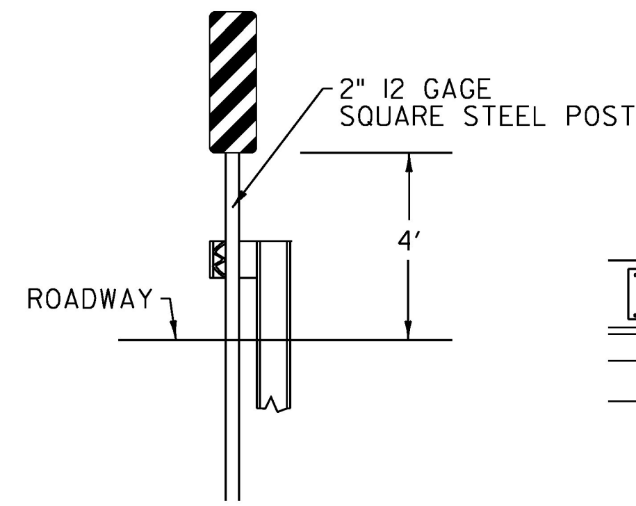
ELEVATION
