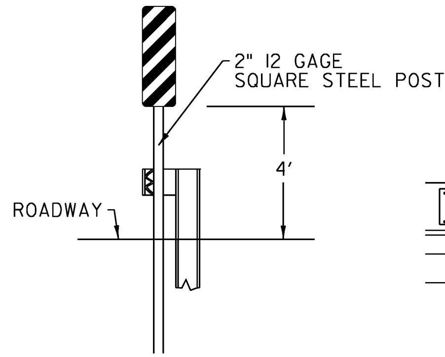
ELEVATION
