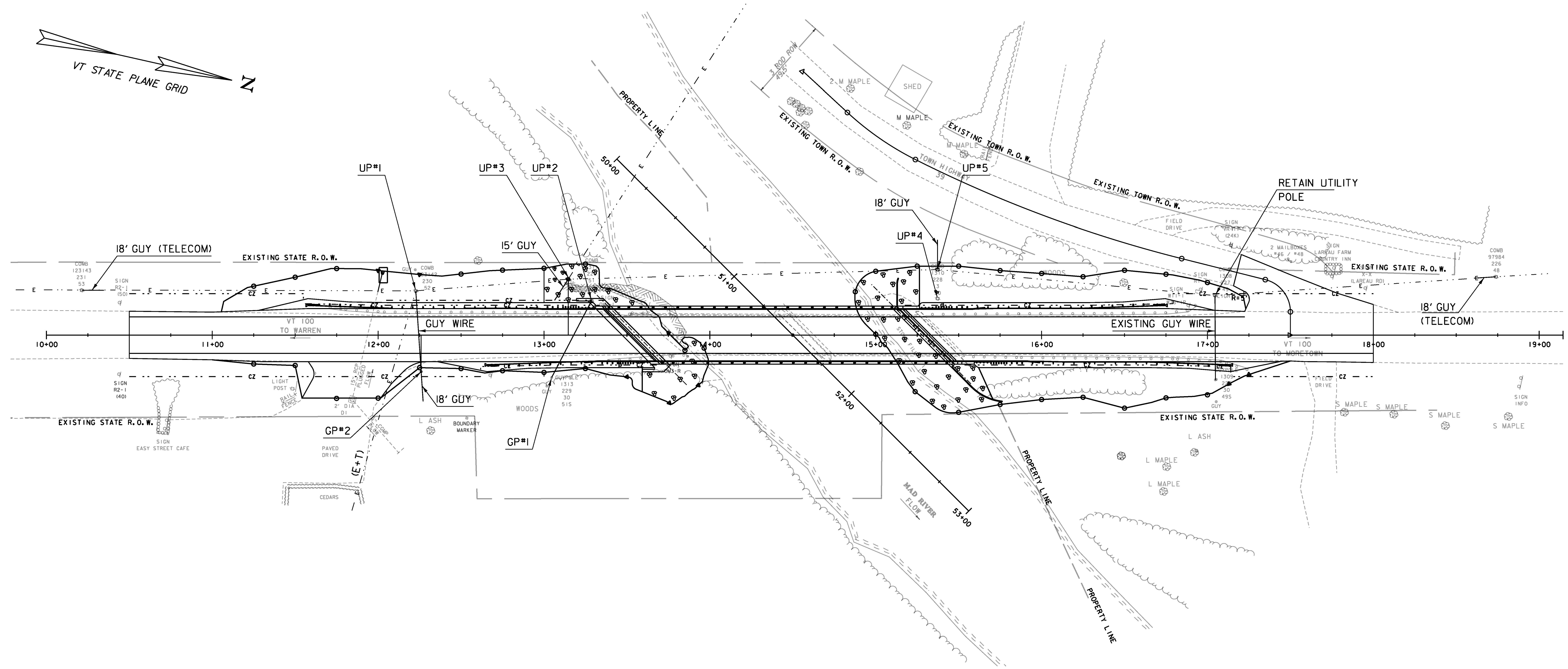
LAYOUT 30 0 30 SCALE: 1" = 30'-0"
