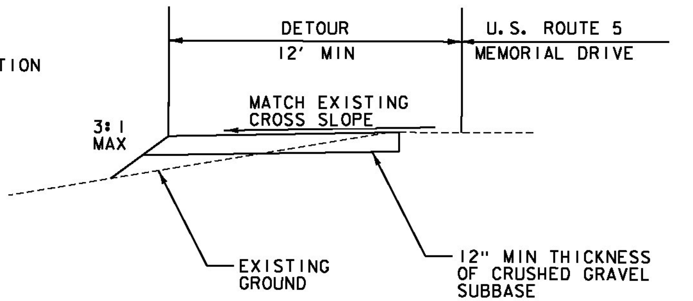
TEMPORARY DETOUR SECTION N. T. S.
