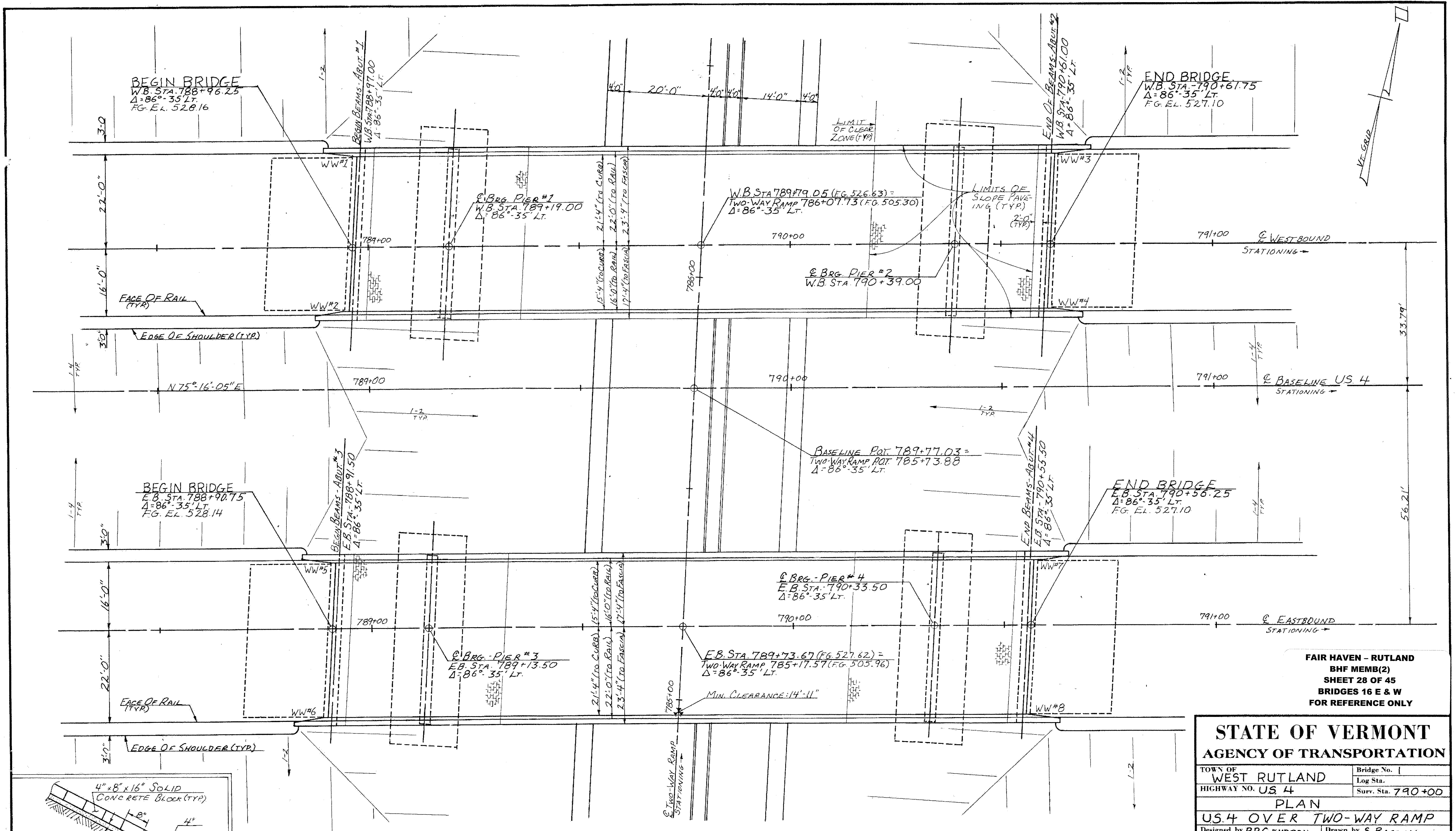
PLAN SCALE: 1" = 10'-0"
