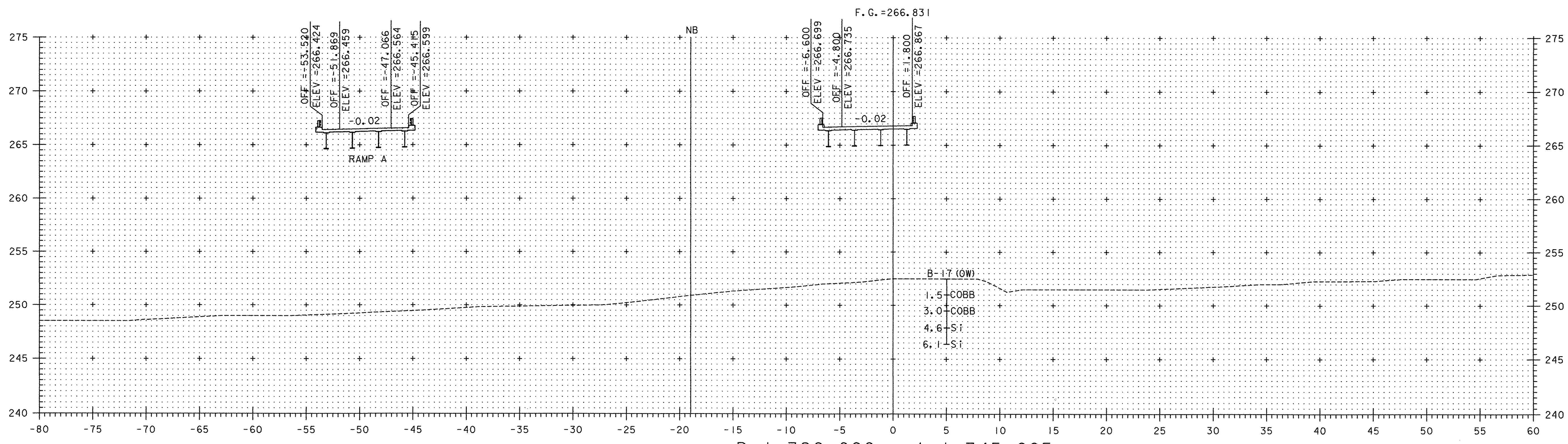
D 1+320.000 = A 1+345.605
