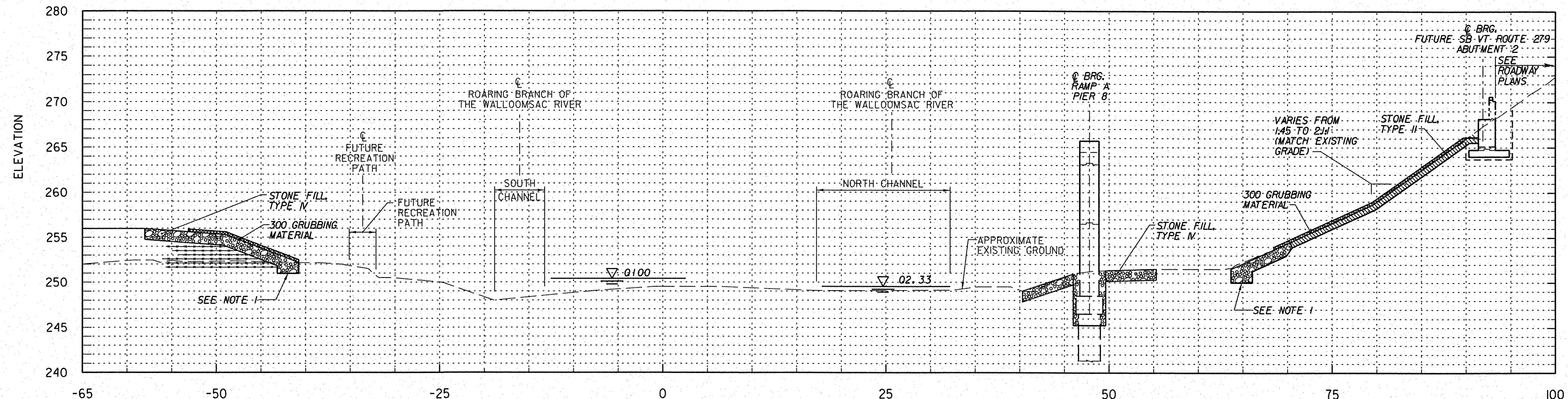
RB 0+140 SCALE 1:250
