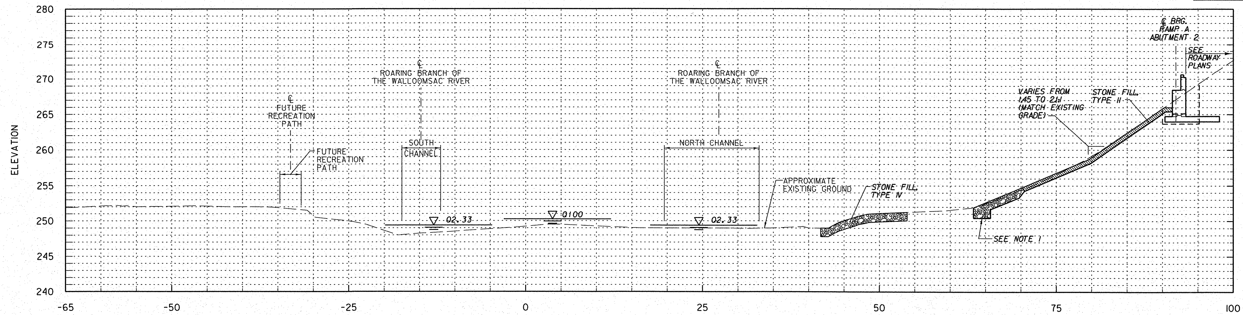
RB 0+145 SCALE 1:250
