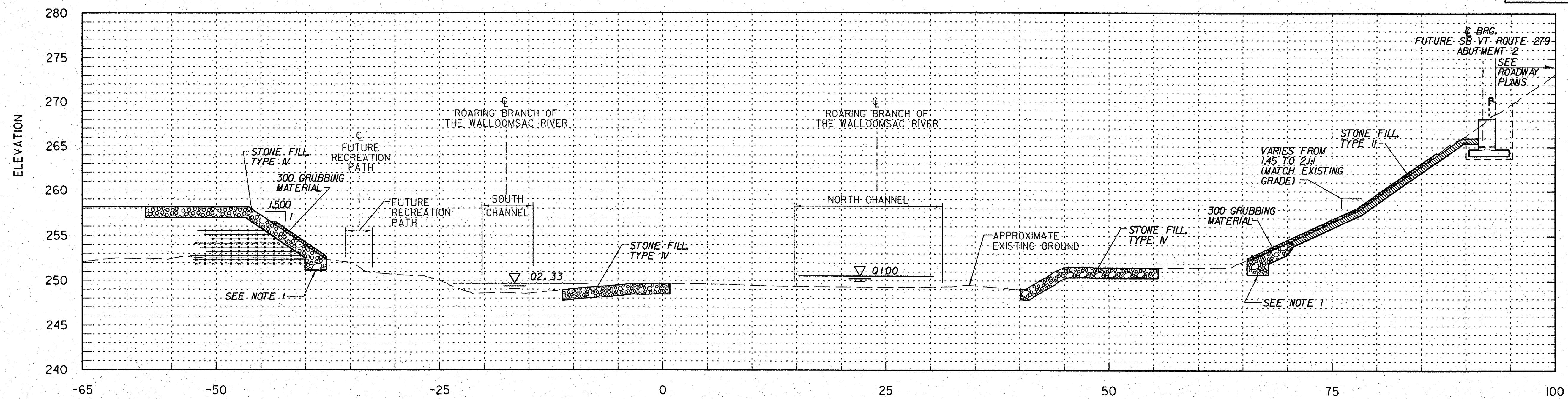
RB 0+135 SCALE 1:250
