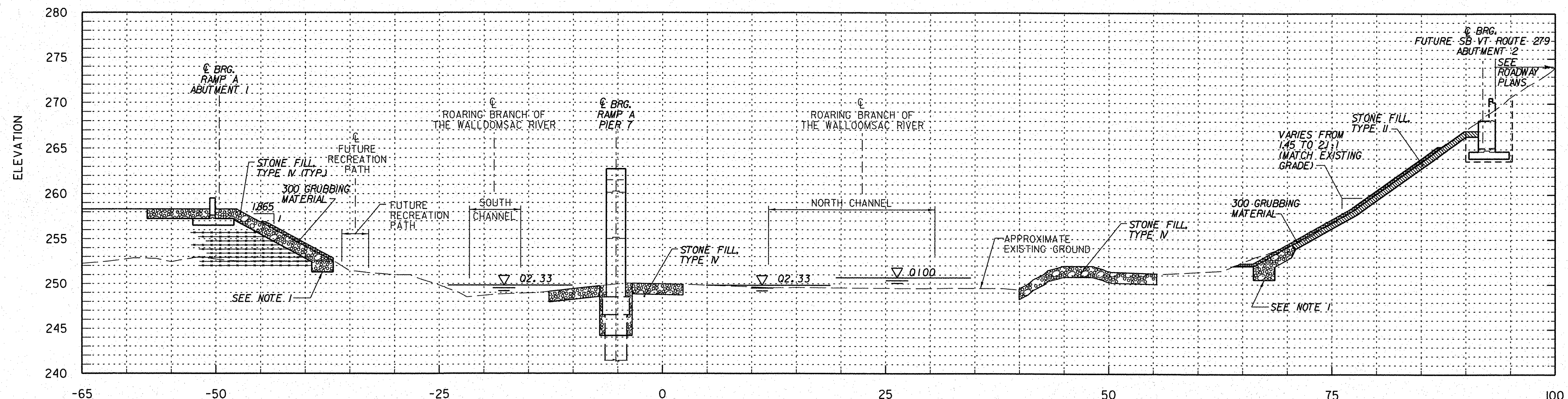
RB 0+130 SCALE 1:250
