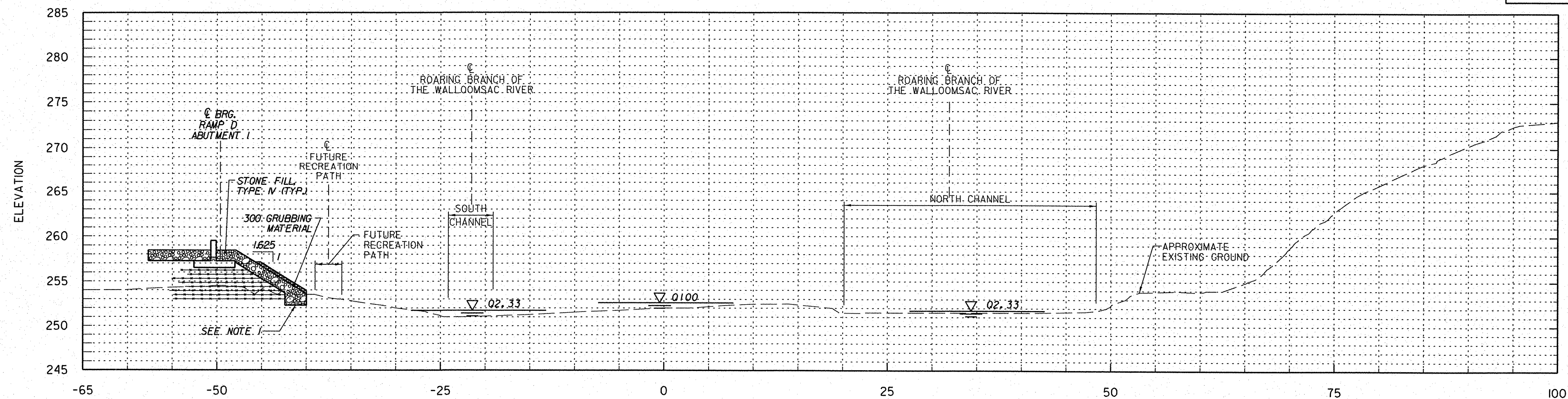
RB 0+065 SCALE 1:250
