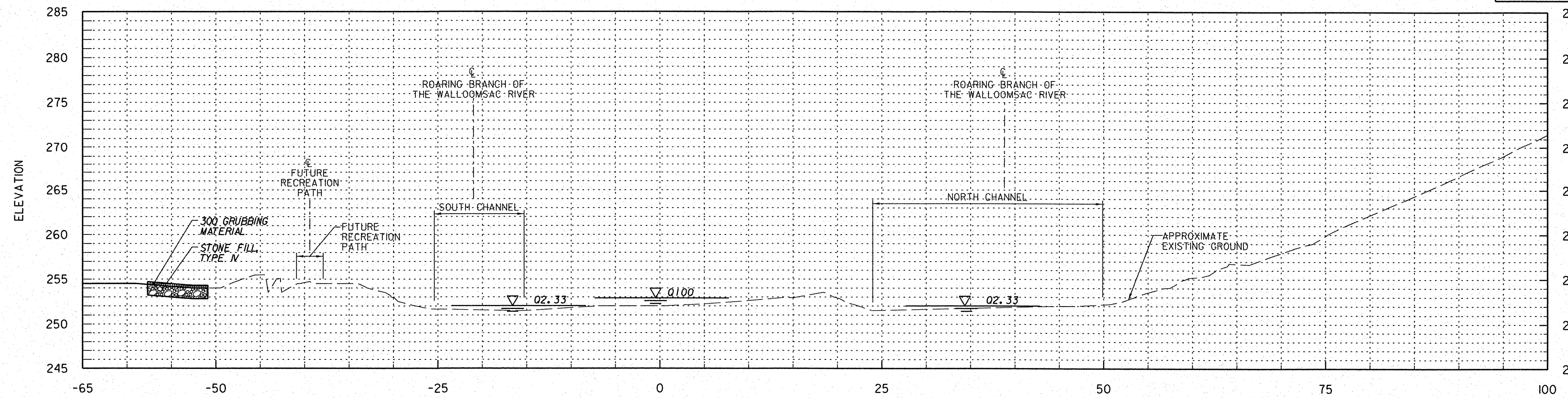
RB 0+055 SCALE 1:250
