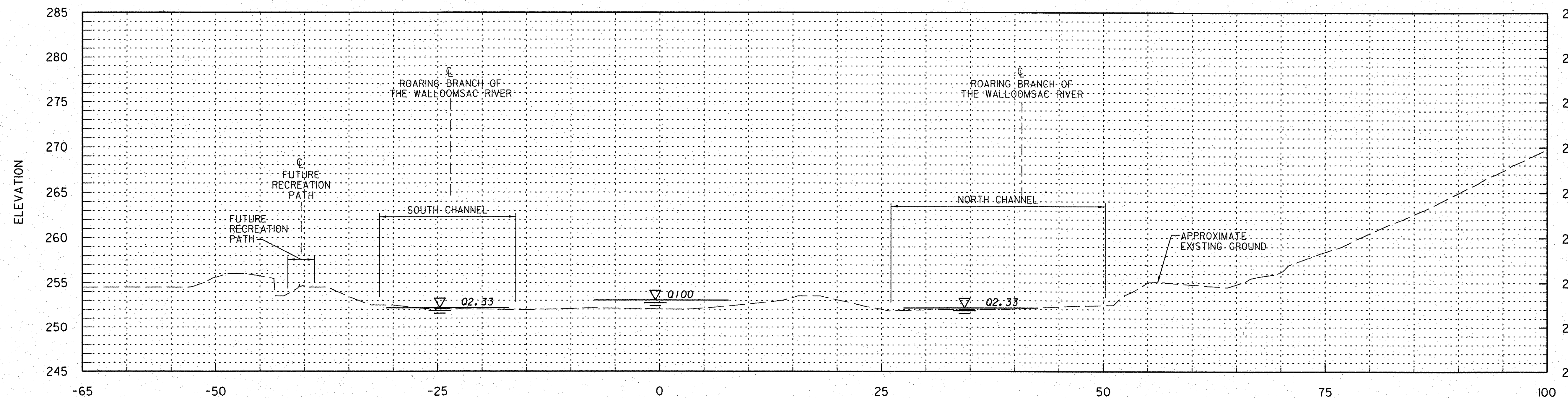
RB 0+050 SCALE 1:250
