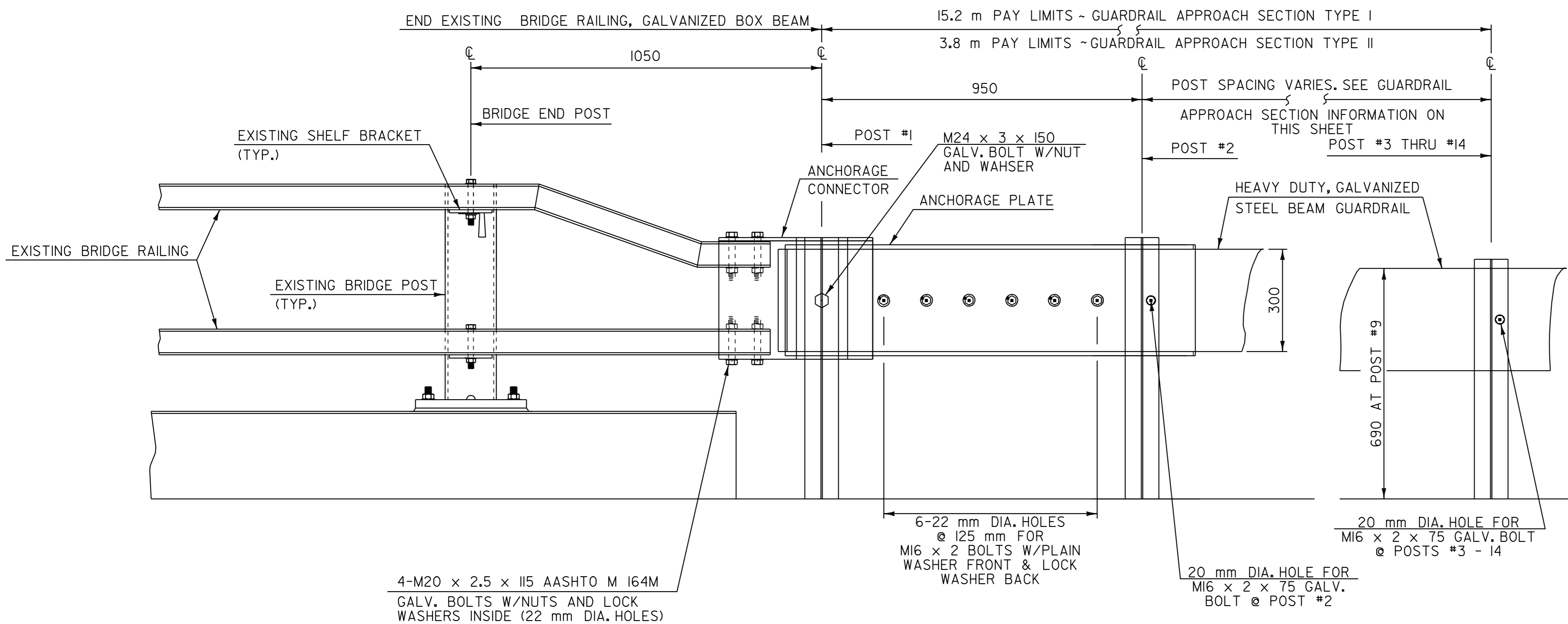
ELEVATION
