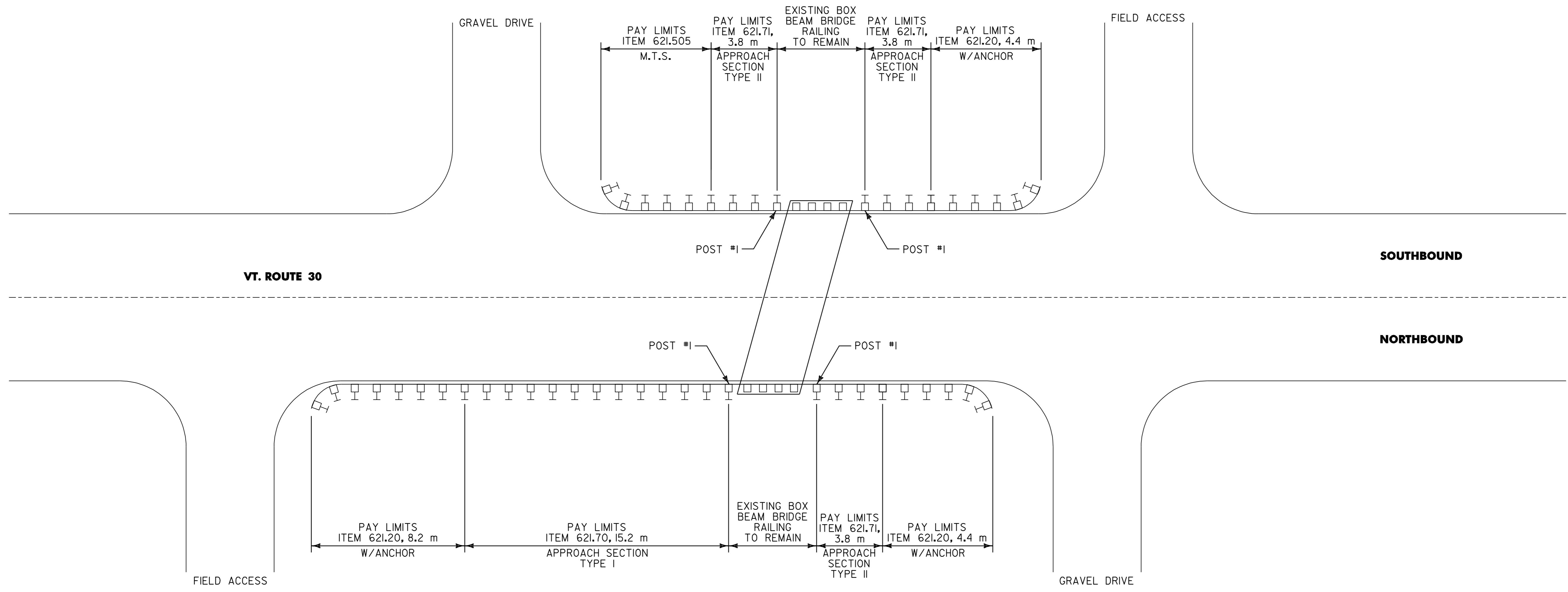
BR 62 RUPERT MM 0.206 = STA. 0+331.525 NOT TO SCALE
