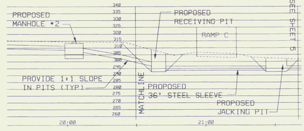
PROFILE SCALE: 1" = 20'
