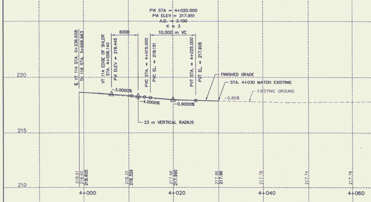
T.H. 118 PROFILE
