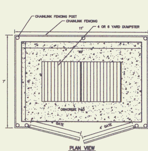
7 DUMPSTER ENCLOSURE DETAILS N.T.S.
