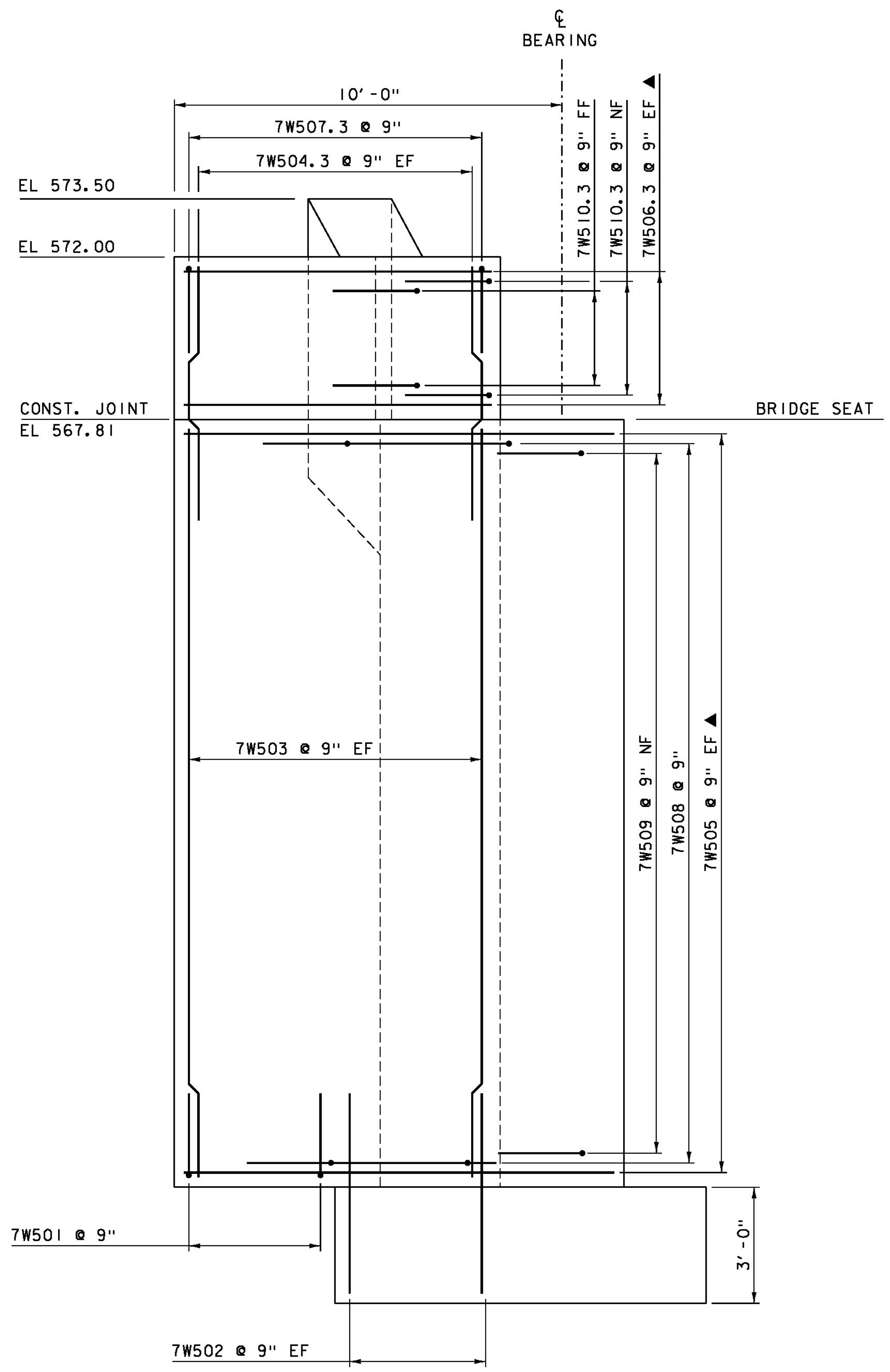
WINGWALL 7 ELEVATION SCALE: 1/2" = 1'-0"
